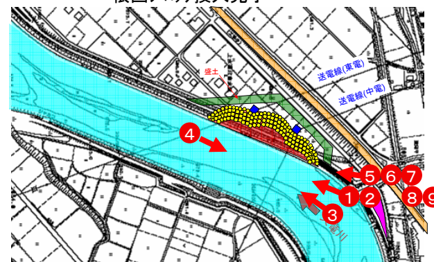
⑥7/24 15時 緊急復旧工事の根固ブロック投入完了
