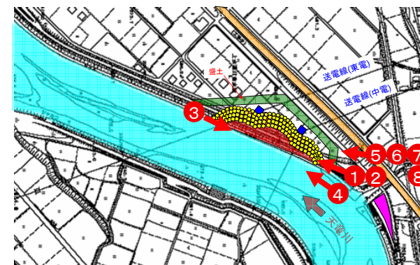
⑥7/26 15時 築堤盛土施工中
