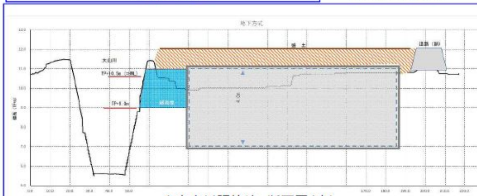
◆大山川調節池 断面図(案)
