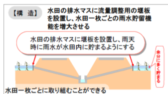
【排水マス流量調整方式】
