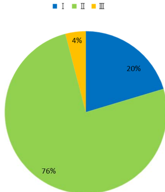
平成26～28年度定期点検結果判定区分 (大型カルバート)
