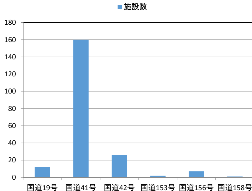
路線別のシェッド数
