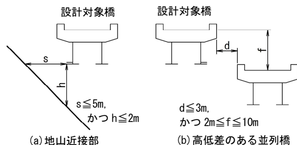
図-5-III-89 腐食の可能性のある箇所
