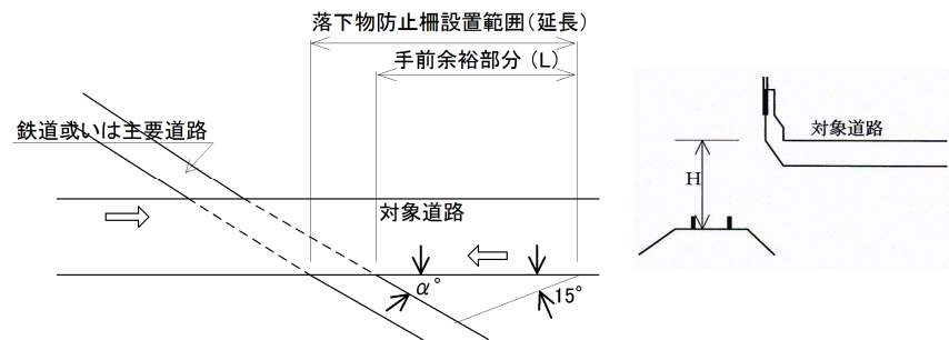
図-5-Ⅲ-77 落下防止柵の設置
