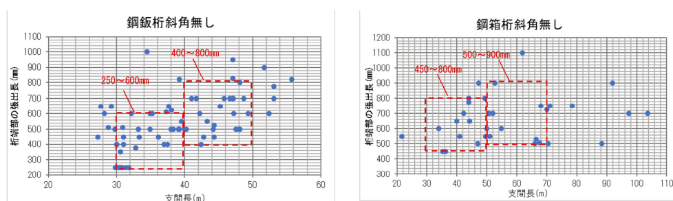
図-5-Ⅲ-10 支間長と桁端部の張出し長さ
