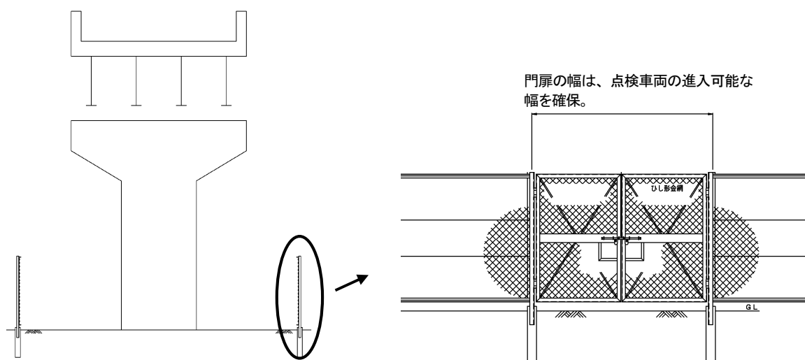
図-5-Ⅲ-123 門扉の設置例
