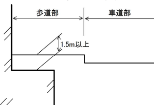
図-5-III-54 フーチングの設置位置
