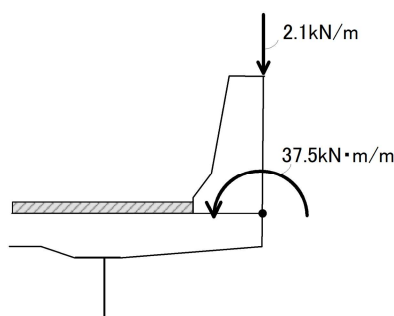
図-5-Ⅲ-1 付属物荷重
