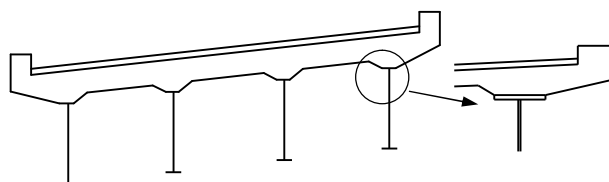
図-5-III-3 鋼板桁の形状
