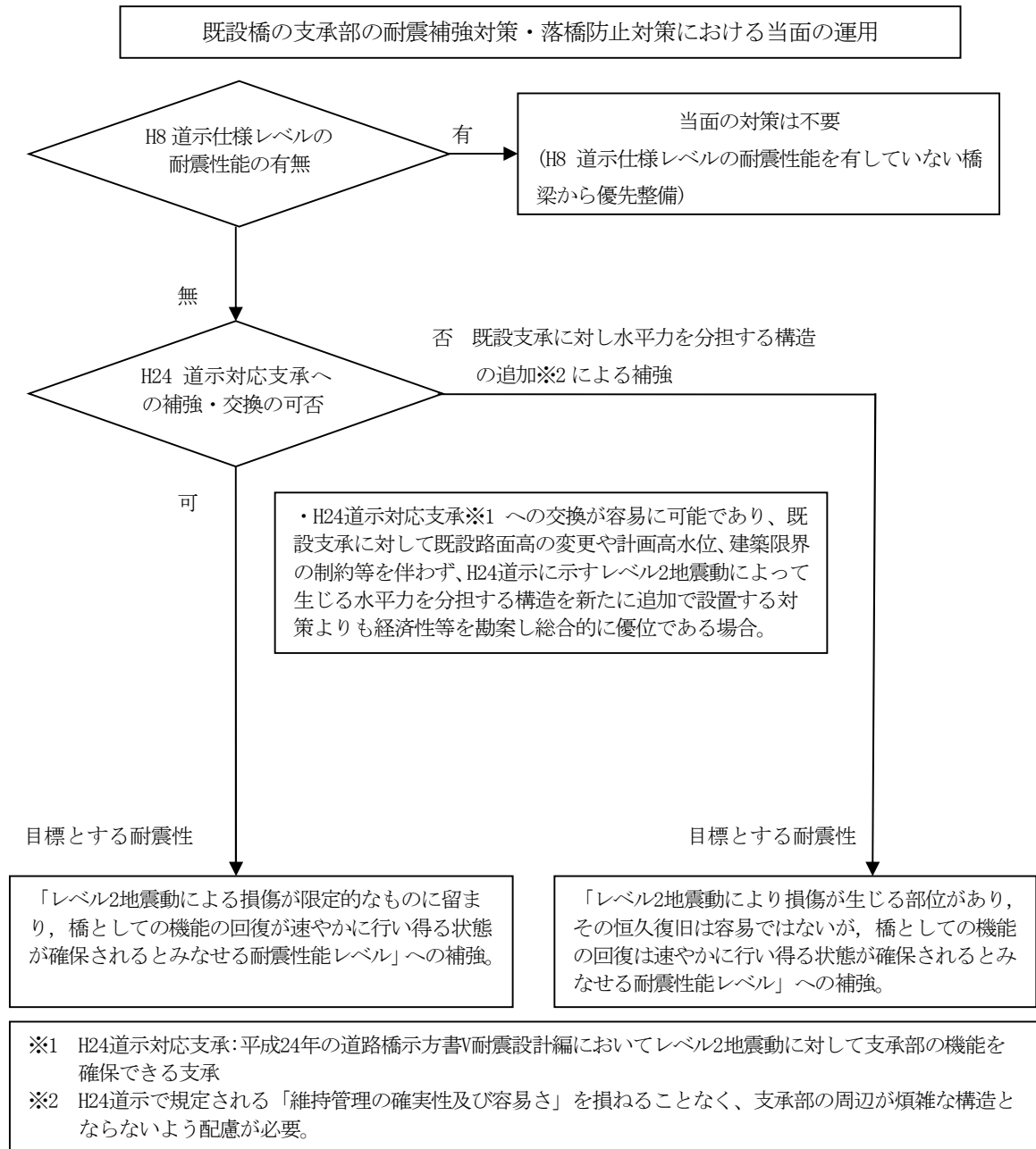
図-5-Ⅲ-124 耐震補強対策・落橋防止対策フロー
