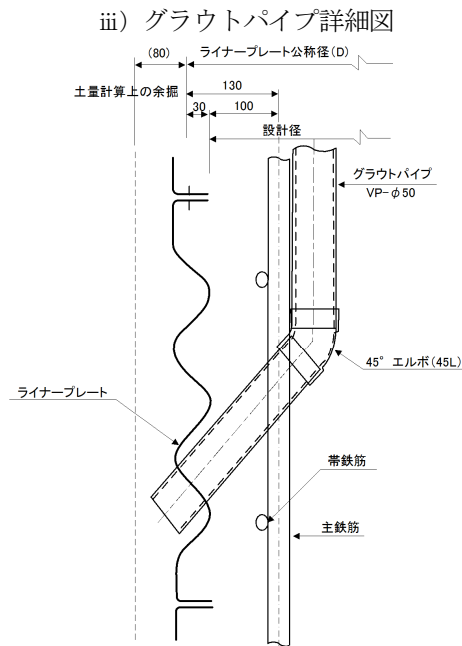
図-5-Ⅲ-62 グラウトパイプ詳細 (参考)
