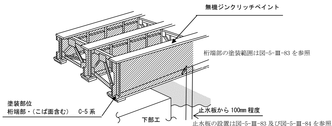
図-5-III-90 保護性さびが形成されにくい箇所の塗装範囲
