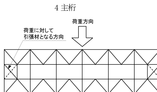
図-5-Ⅲ-12 直橋 (4 主桁)
