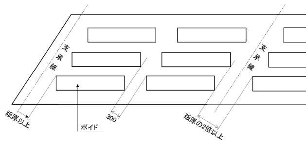
図-5-Ⅲ-38 横桁の厚さ
