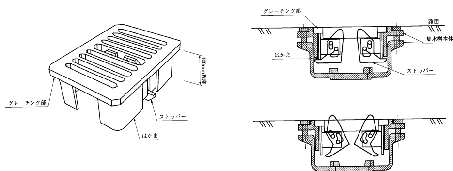
図-5-III-72 排水枥（参考）
