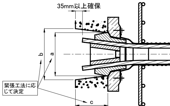
図-5-Ⅲ-100 PC鋼材定着部切り欠きの例
