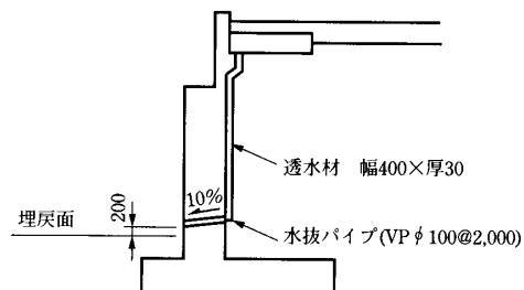
図-5-Ⅲ-51 橋台背面処理
