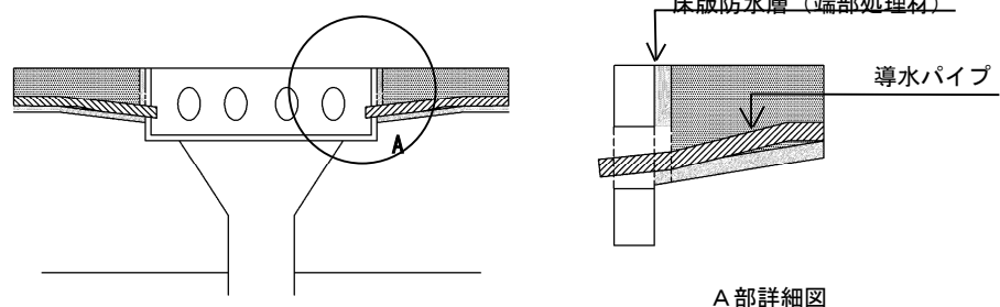
図-5-Ⅲ-113 伸縮装置付近の防水層立ち上げの例
