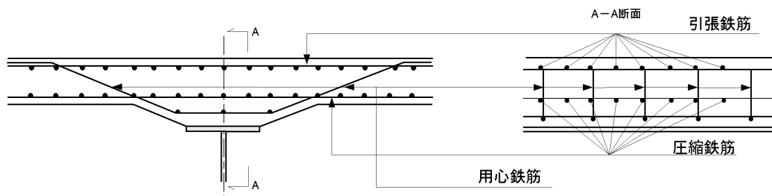
図-5-Ⅲ-26 ハンチの標準構造及び用心鉄筋の配置
