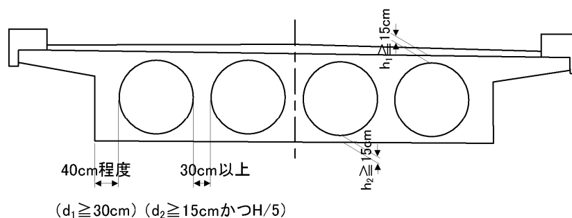
図-5-III-36 PC 中空床版橋の断面形状（標準値）
