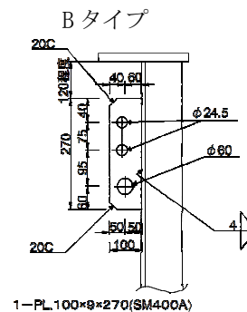
図-5-Ⅲ-23 B タイプ
