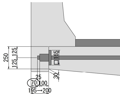
図-5-Ⅲ-101 定着部のかぶりを70mmとした例
