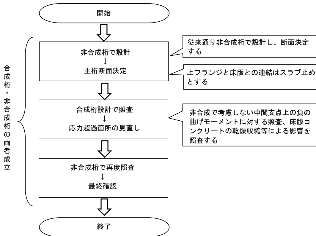
図-5-Ⅲ-8 コンクリート系床版を有する鋼桁の設計フロー（参考）
