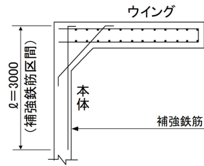
図-5-Ⅲ-49 パラペット本体の補強
