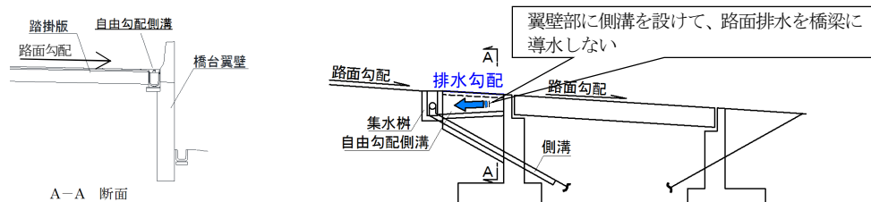
図-5-Ⅲ-79 周辺地形から橋に水が集まらない構造及び排水の計画の例
