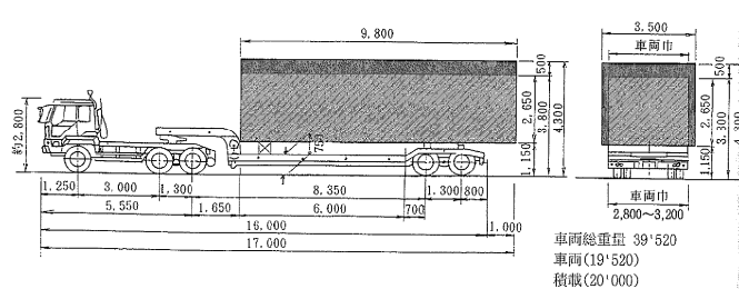
図-5-Ⅲ-7 低床式セミトレーラー輸送姿図
