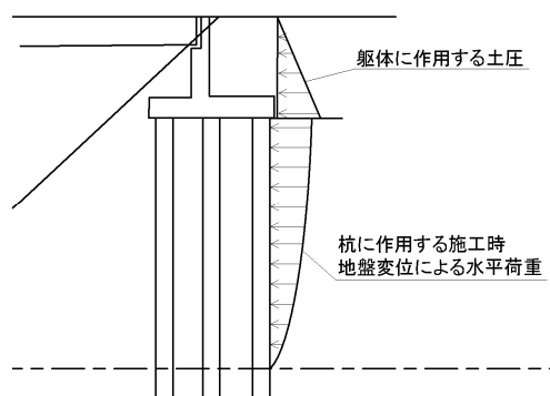
図-5-II-5 盛りこぼし橋台のイメージ
