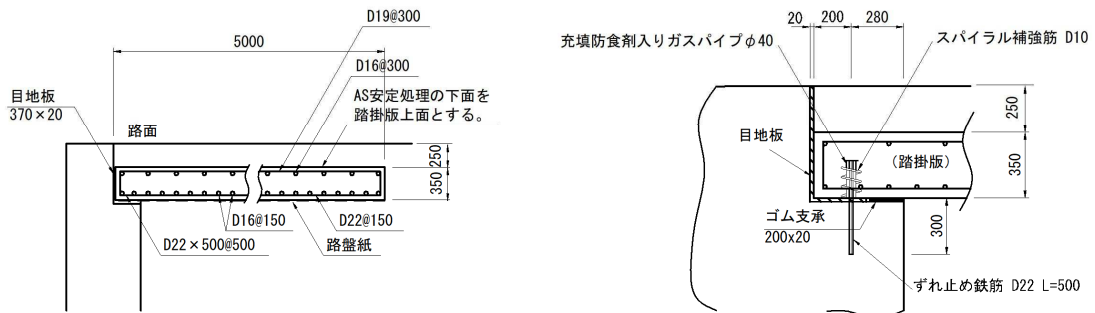
図-5-Ⅲ-50 踏掛版の構造（参考）
