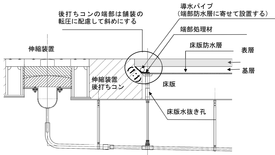
図-5-Ⅲ-113 伸縮装置付近の防水層立ち上げの例
