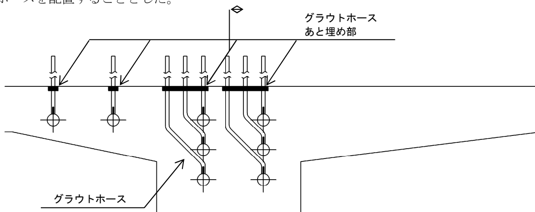
図-5-III-105 グラウトホースのあきの例
