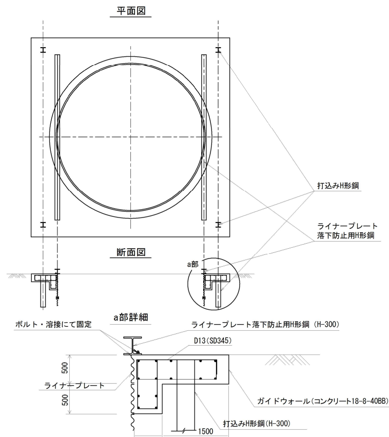
図-5-Ⅲ-63 ガイドウォールの沈下対策 (参考)
