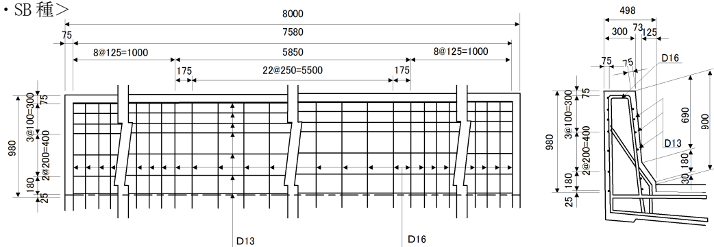
図-5-III-64 壁高欄（剛性防護柵）の配筋
