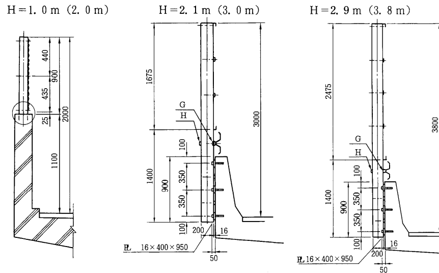
図-5-Ⅲ-76 落下物防止柵の形状
