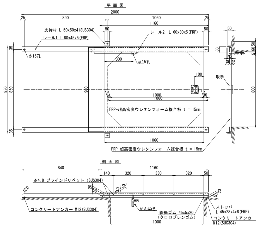
図-5-Ⅲ-108 マンホール蓋の例
