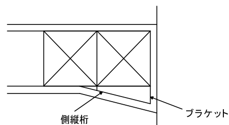
(b) 側縦桁配置
