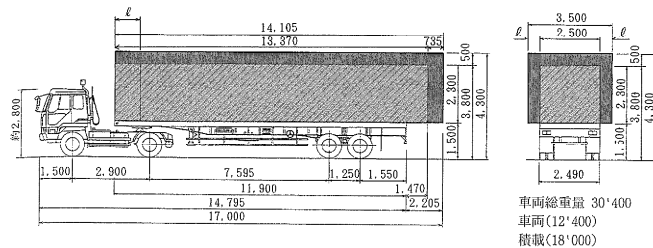
図-5-Ⅲ-6 高床式セミトレーラー輸送姿図
