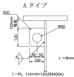
図-5-Ⅲ-22 A タイプ
