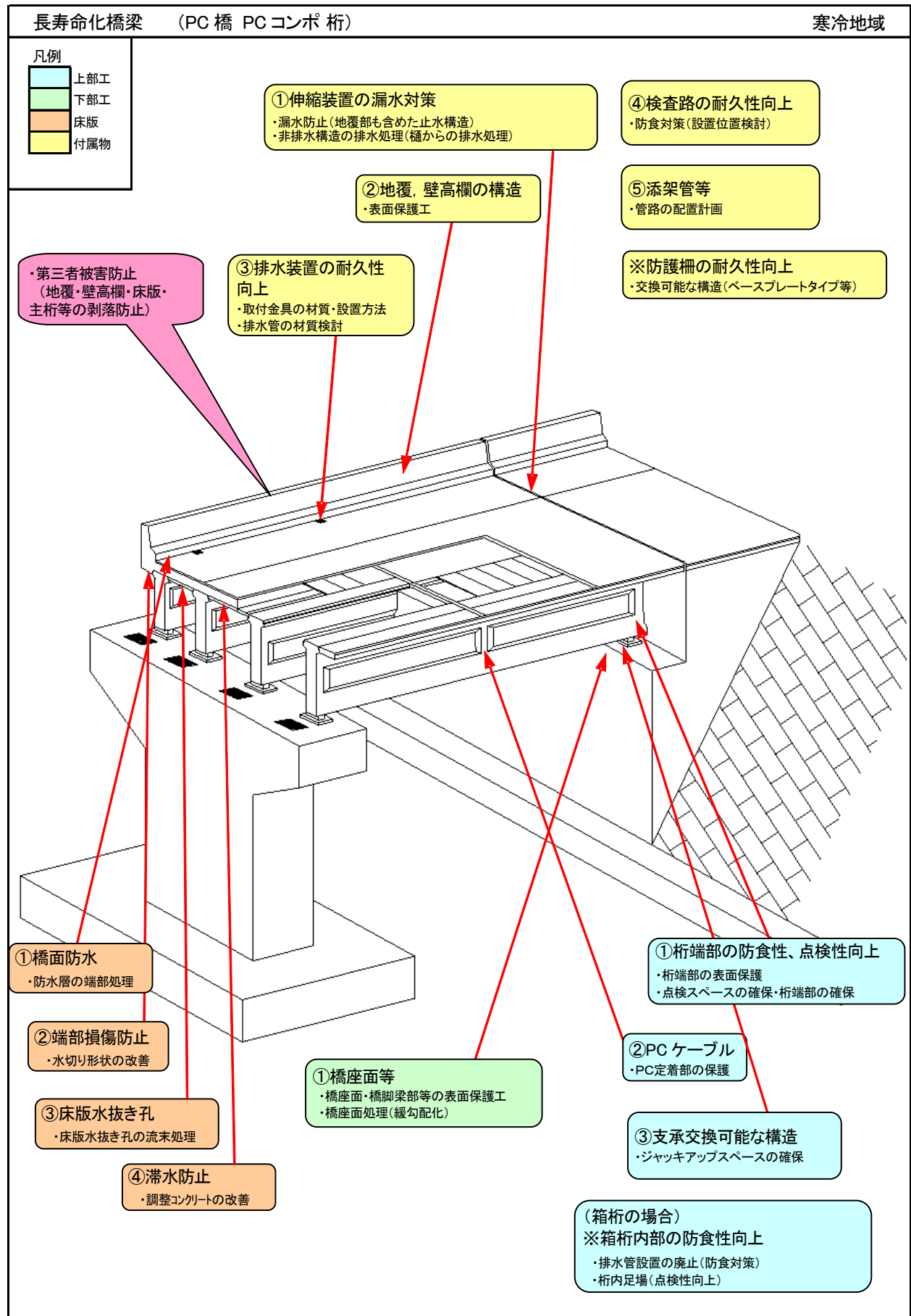
図-5-Ⅲ-81 PC 橋の主な長寿命化対策項目例
