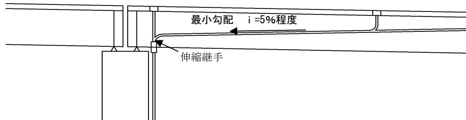
図-5-III-118 排水管の勾配
