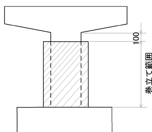
図-5-Ⅲ-126 梁下の処理
