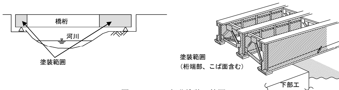
図-5-Ⅲ-88 部分塗装の範囲
