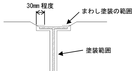
図-5-Ⅲ-86 まわし塗装の範囲
