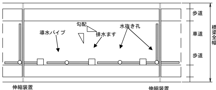
図-5-Ⅲ-115 排水資材の配置例
