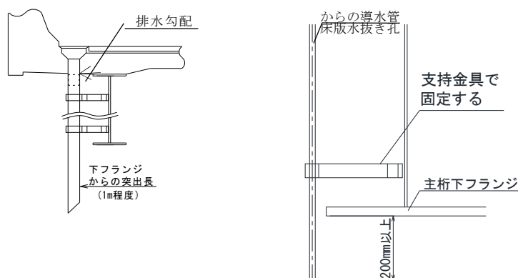
図-5-III-85 排水構造の吐け口と主桁の高さ関係
