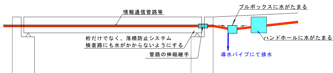
図-5-Ⅲ-122 添架物等の配管部を伝い橋梁部への漏水を防止する構造例
