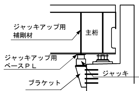
図-5-Ⅲ-98 下部工付ブラケット仮受工法による 支承取替え
