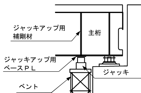
図-5-Ⅲ-97 ベントによる仮受工法による支承取替え
