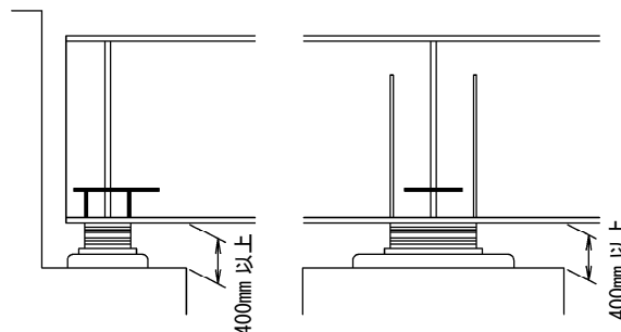
図-5-III-110 桁下空間
