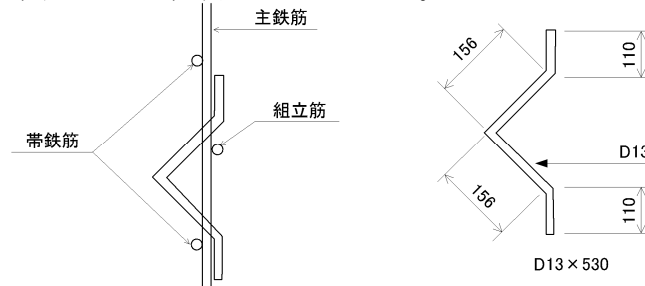
図-5-Ⅲ-58 スペーサー形状(参考)
