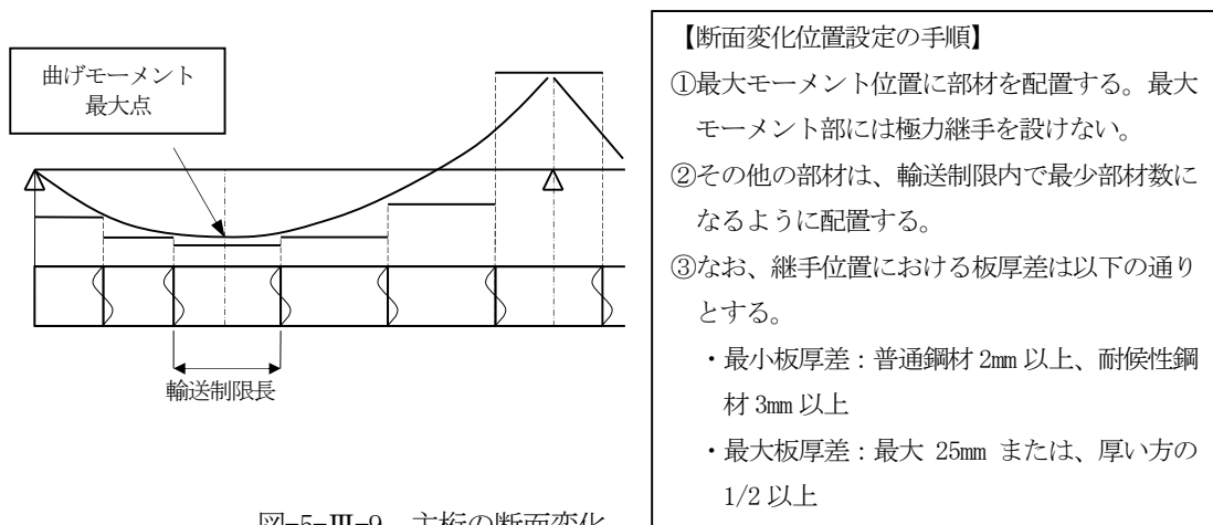
図-5-Ⅲ-9 主桁の断面変化
