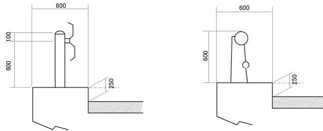
図-5-III-67 支柱式車両用防護柵（参考）
