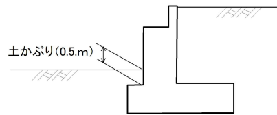
図-5-Ⅲ-56 フーチングの土かぶり
