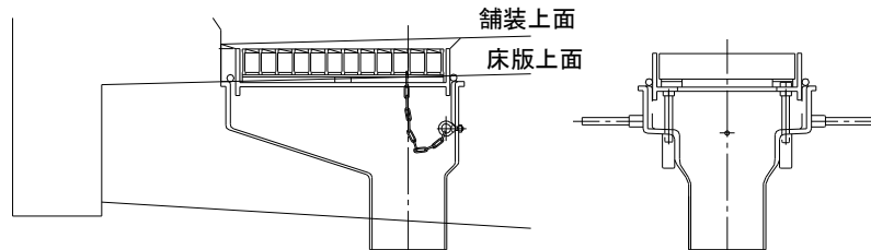
図-5-Ⅲ-120 排水ます (FRP) の例
