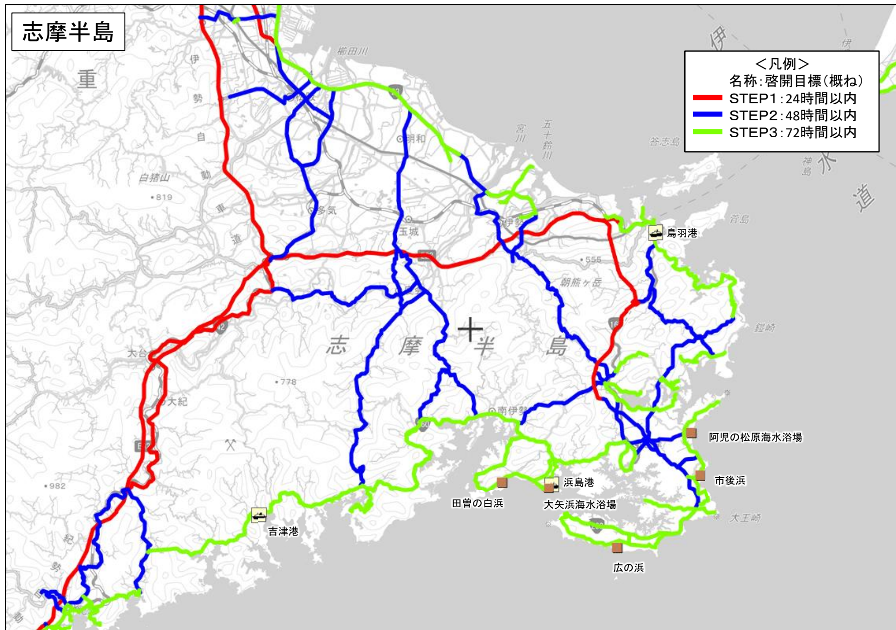
図4-7 志摩半島における港湾・砂浜位置図
