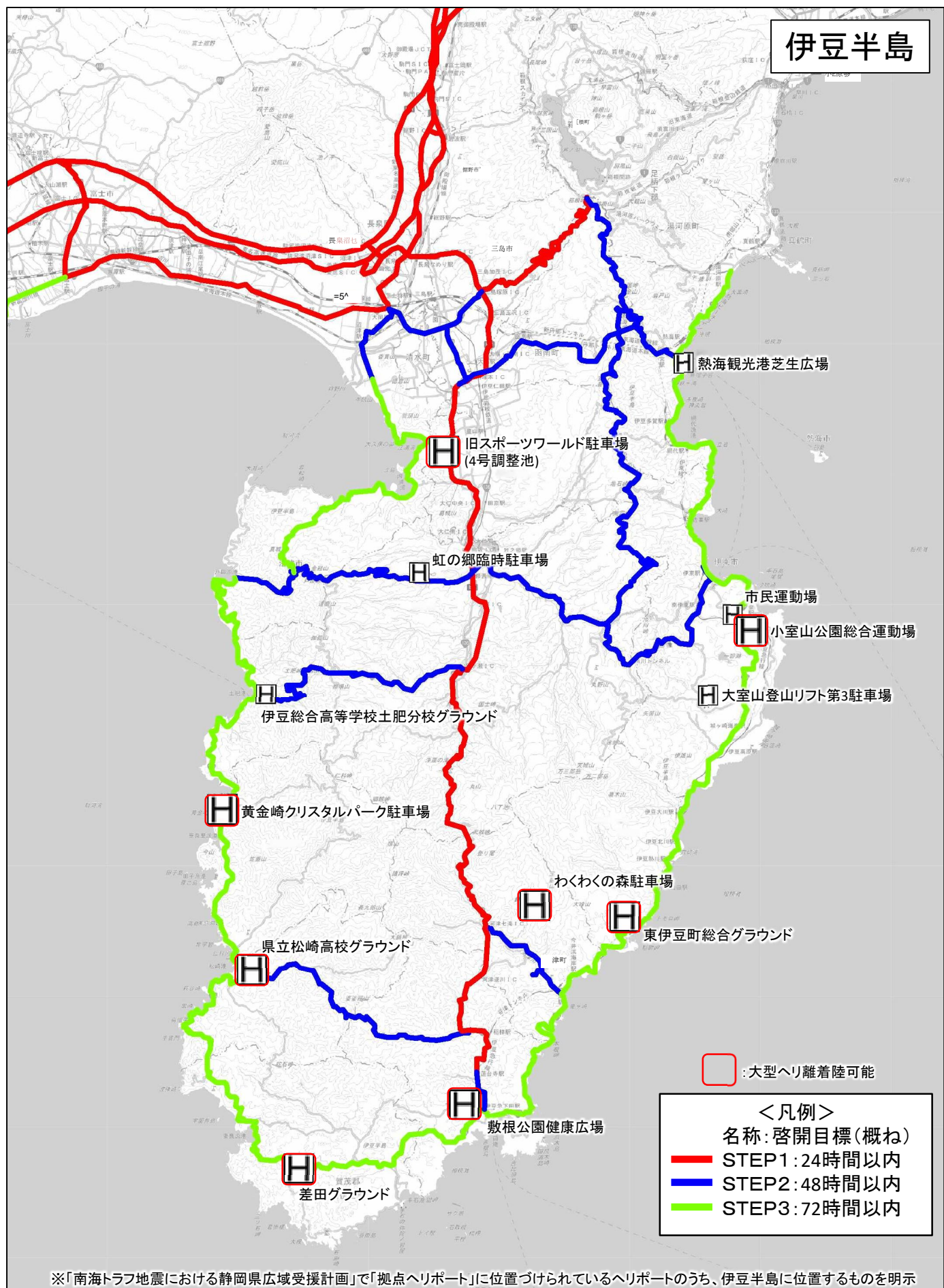
別図4-1 伊豆半島におけるヘリポート位置図
