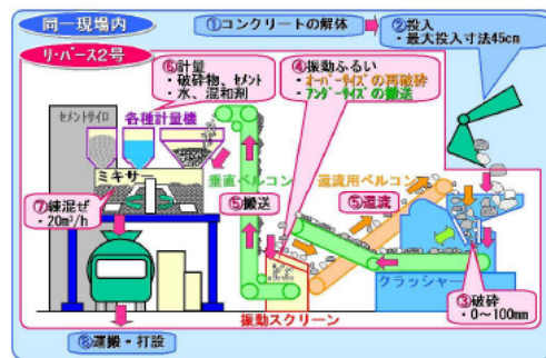
図-1 製造方法のイメージ (2号機)
