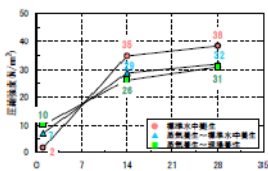
図-3 圧縮強度
