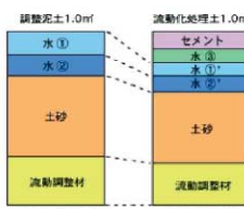
■混練り時の配合設定模式図
