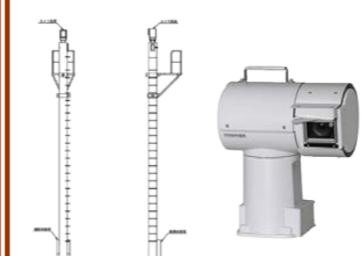
【カメラ支柱姿図(参考)】
