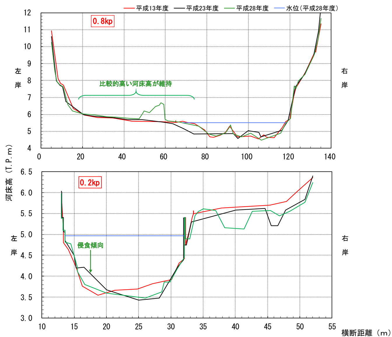
図 2-6 横断形状の経年変化
