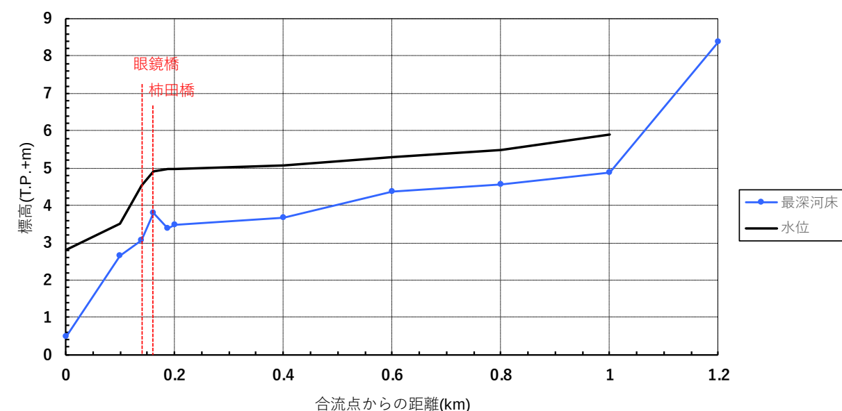
図 1-6 柿田川の縦断形状（2016 年度縦横断測量結果）
