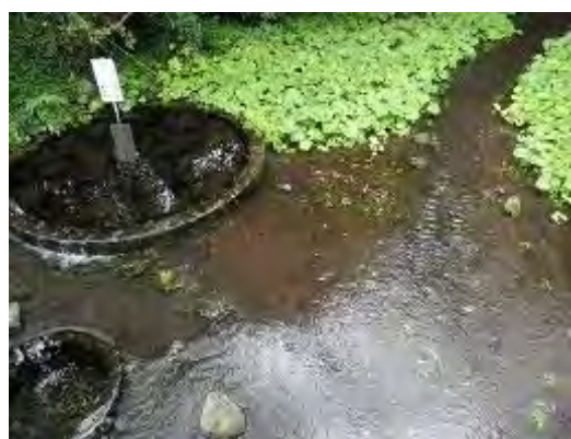
アユ産卵場の状況
