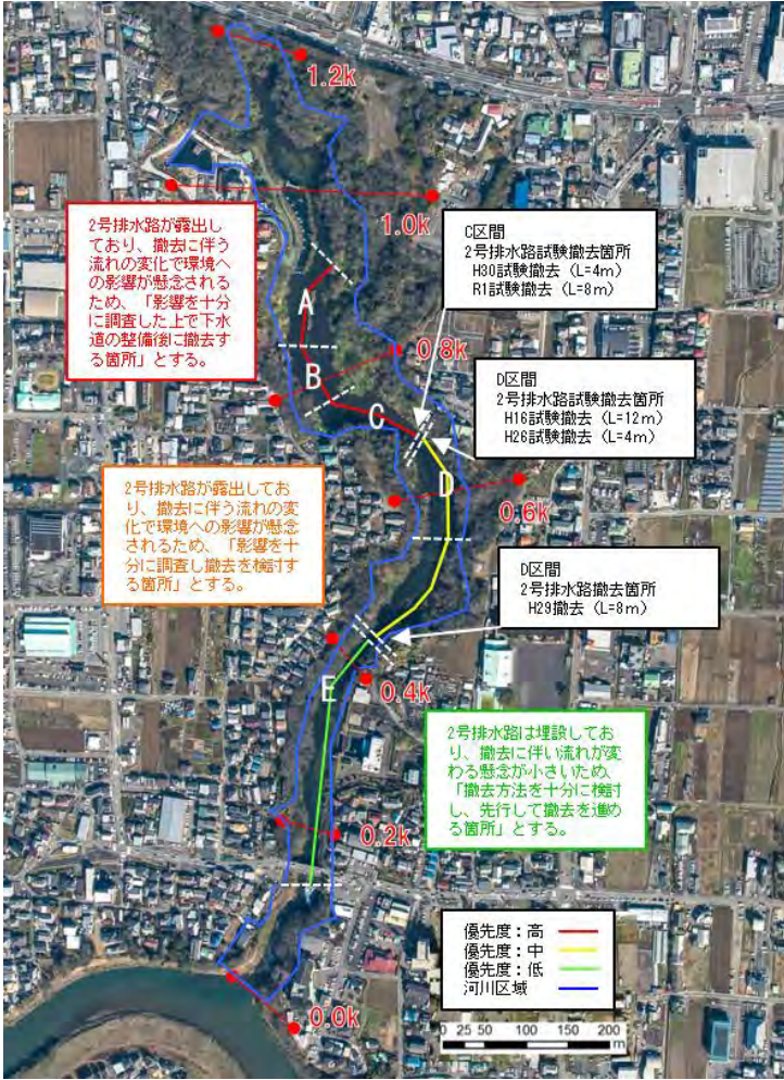
図 5-7 2号排水路撤去のための事前評価及び方針検討に係る整備箇所
