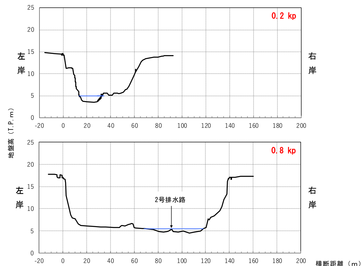
図 1-7 柿田川の横断形状（2016 年度縦横断測量結果）
