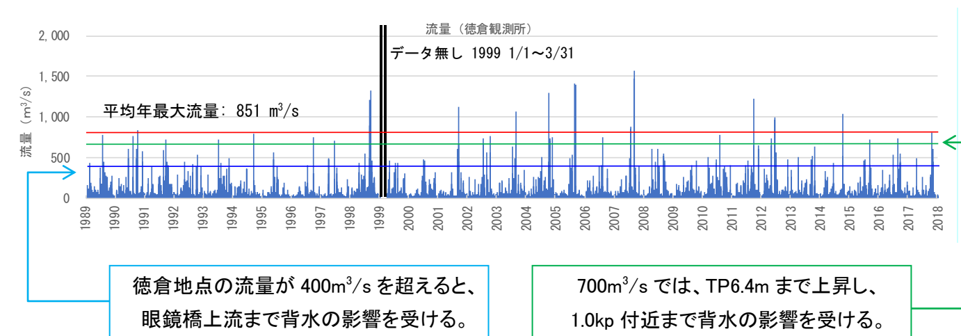
図 1-8 狩野川本川の出水による柿田橋への背水
