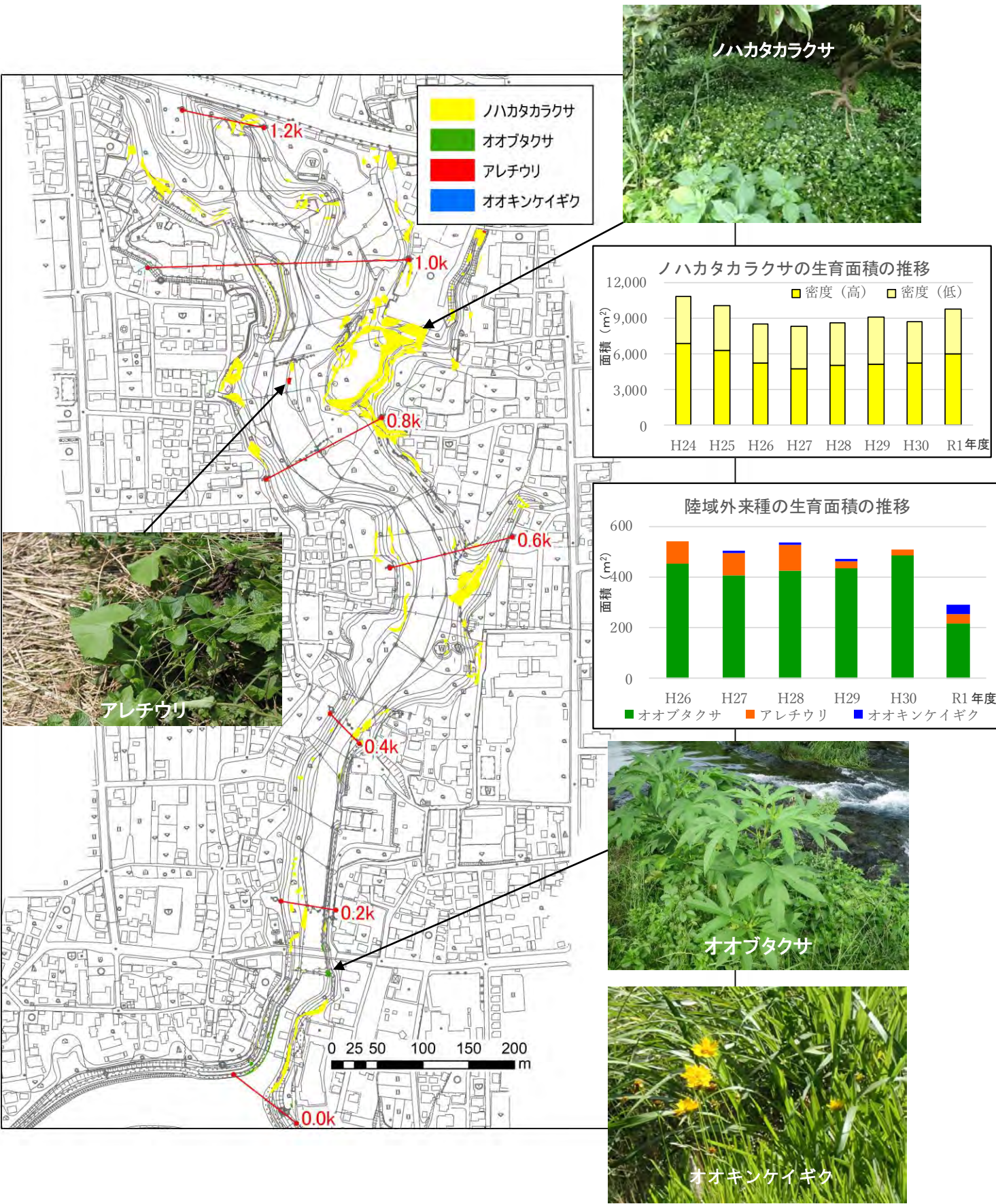
図2-11 ノハカタカラクサ、オオブタクサ、アレチウリ、オオキンケイギクの生育状況
