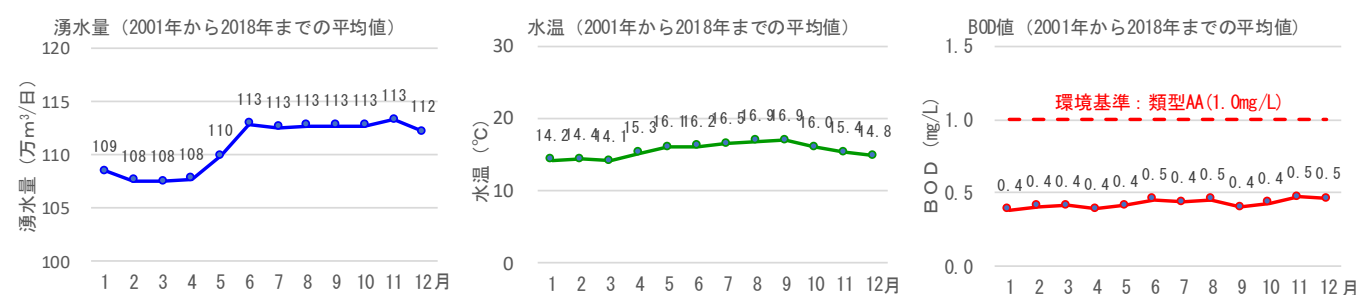
図 1-5 柿田川の湧水量・水温・BOD 値の経月変化（柿田橋）
