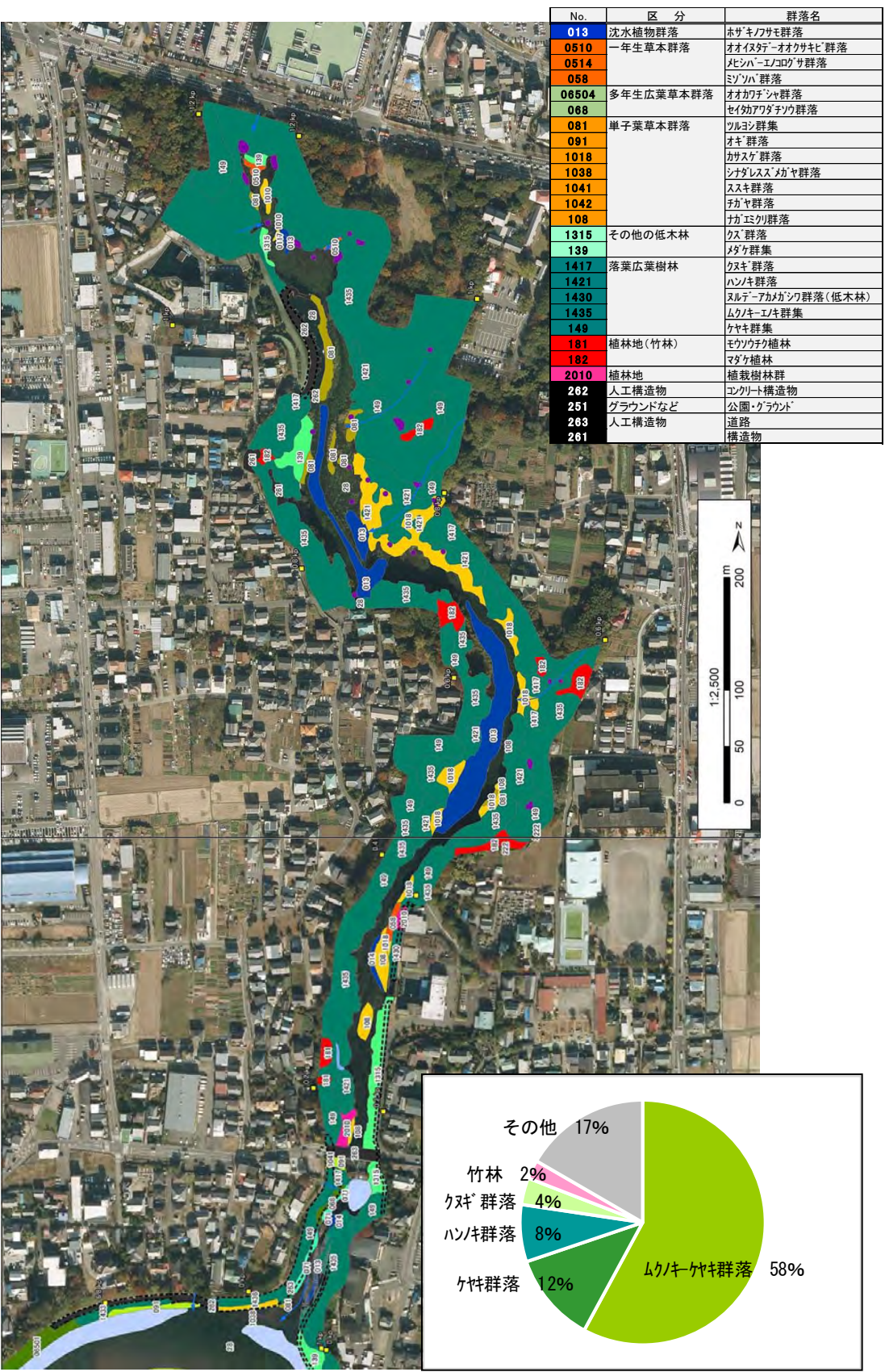
図 1-10 陸域植生の状況 （植生図は、2018 年度狩野川河川水辺環境調査による）
