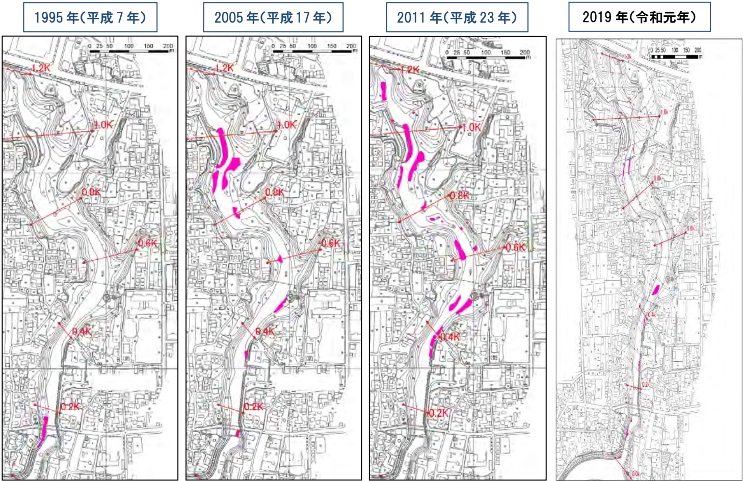
図2-10 ツルヨシ生育状況の変化
