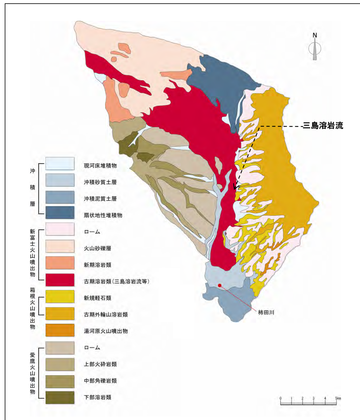
図 1-2 地質集成図
