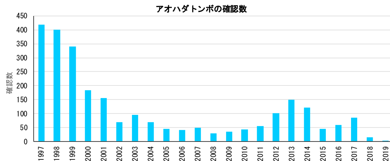
図 2-13 アオハダトンボの確認状況 ※データ提供：(公財)柿田川みどりのトラスト
