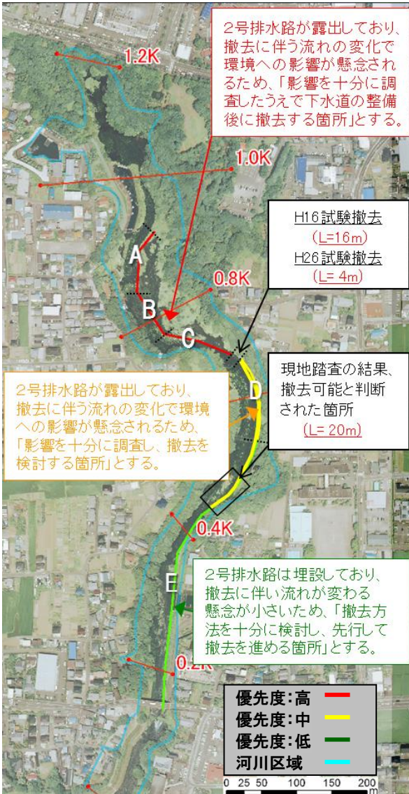
図 5-7 2号排水路撤去のための事前評価及び方針検討に係る整備箇所
