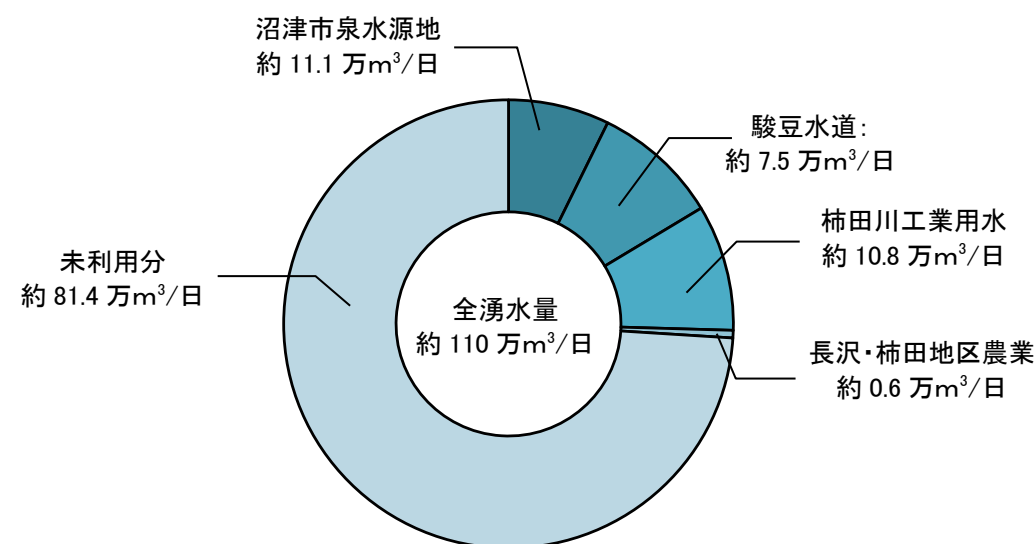
図 1-11 柿田川水利用の状況
