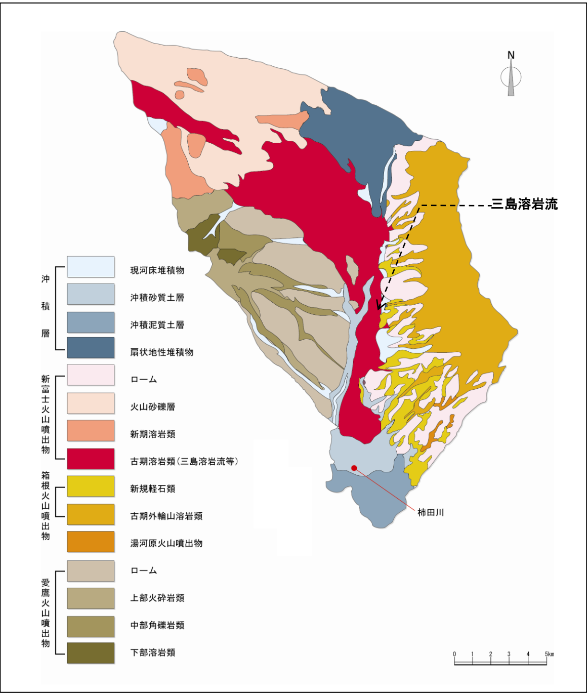
図 1-2 地質集成図
