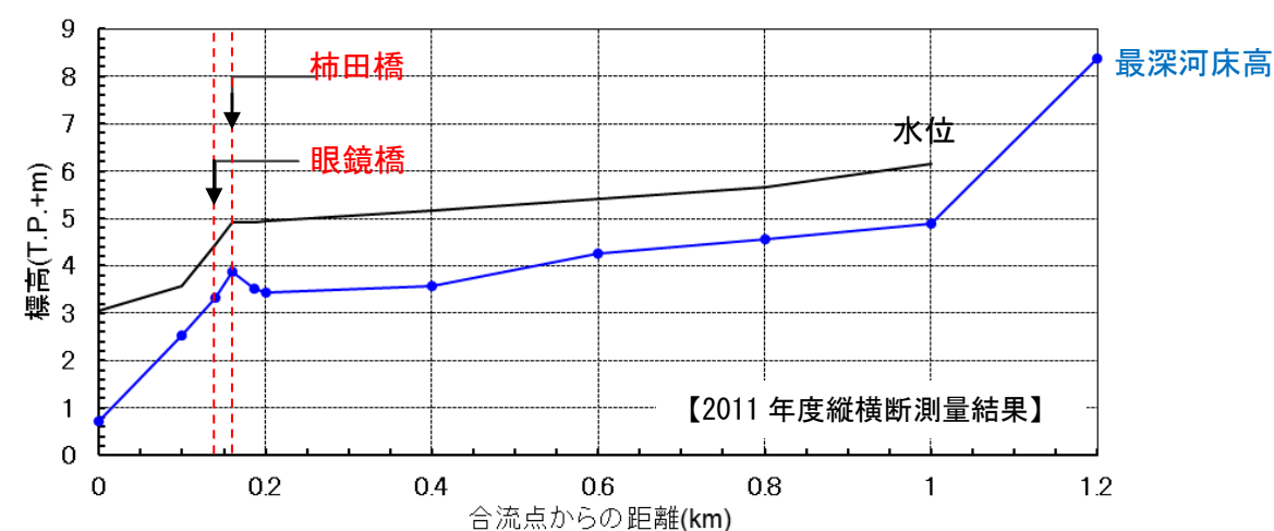
図 1-6 柿田川の縦断形状
