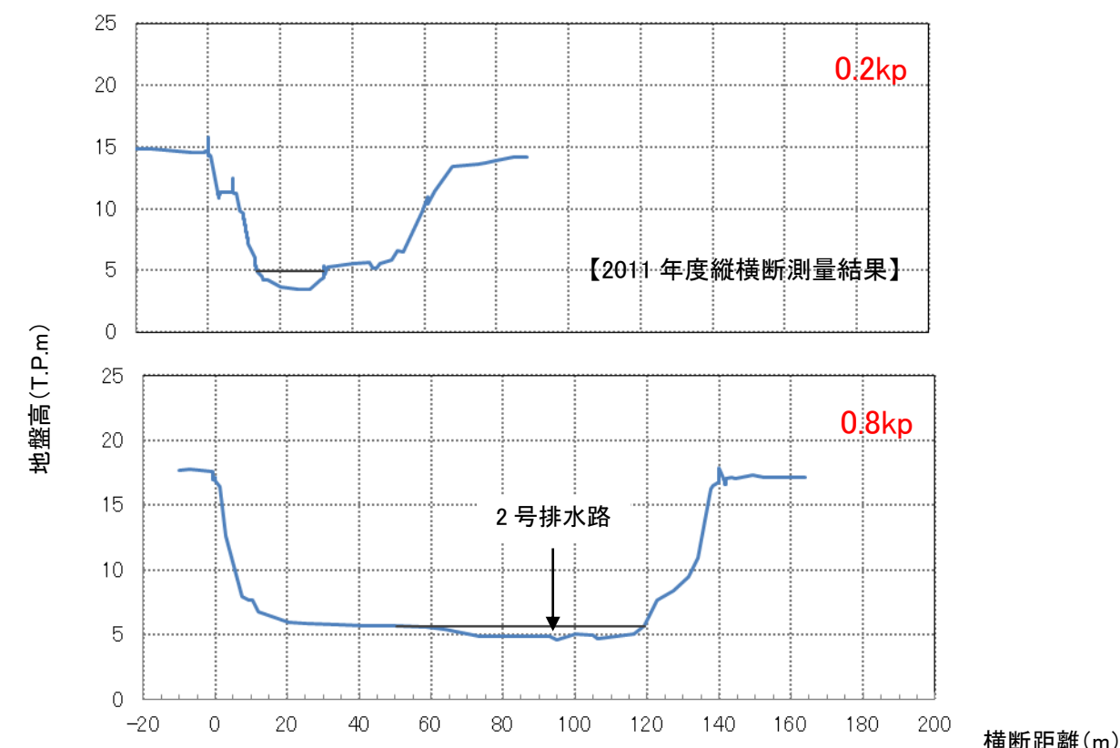
図 1-7 柿田川の横断形状
