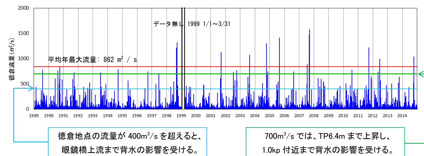
図 1-8 狩野川本川の出水による柿田橋への背水
