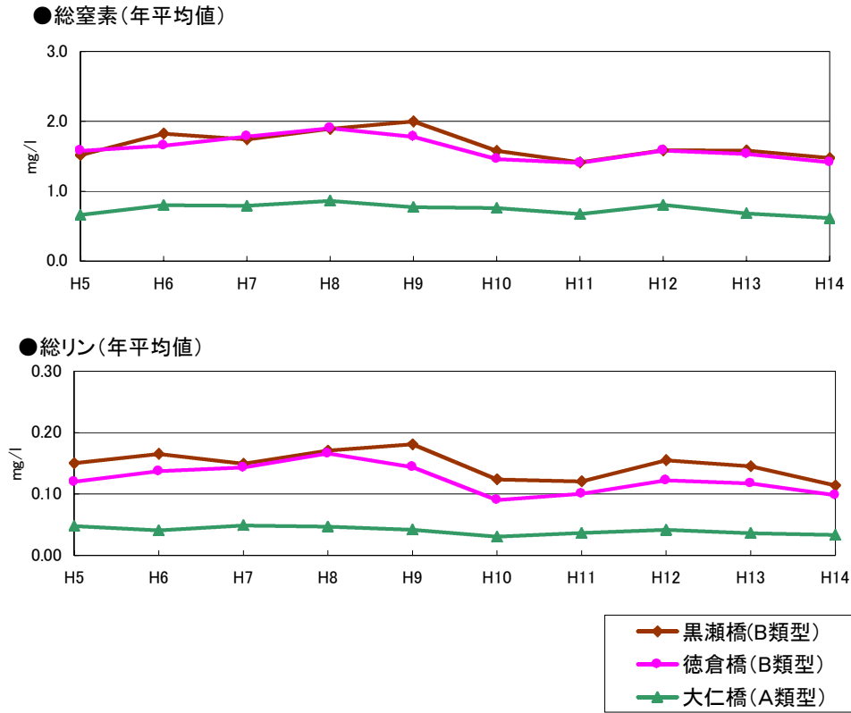
図2.1.7(2) 狩野川本川環境基準地点における水質
