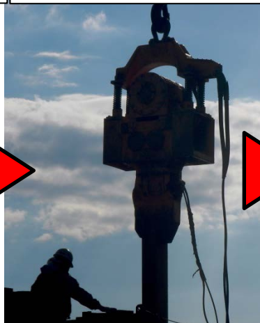
電動式パイフロハンマ により鋼矢板を打ち込み
