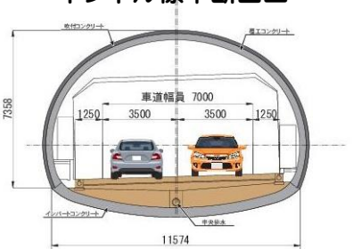
トンネル標準断面図
