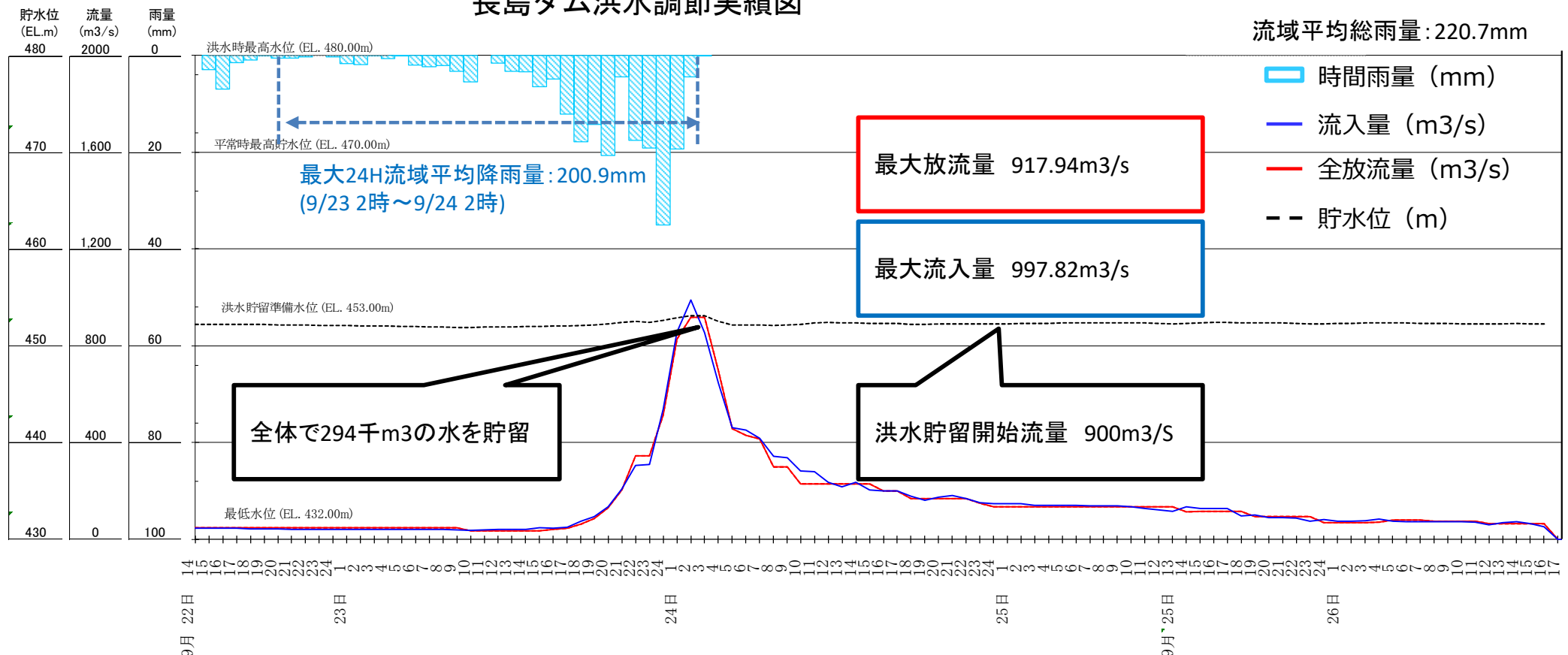
長島ダム洪水調節実績図
