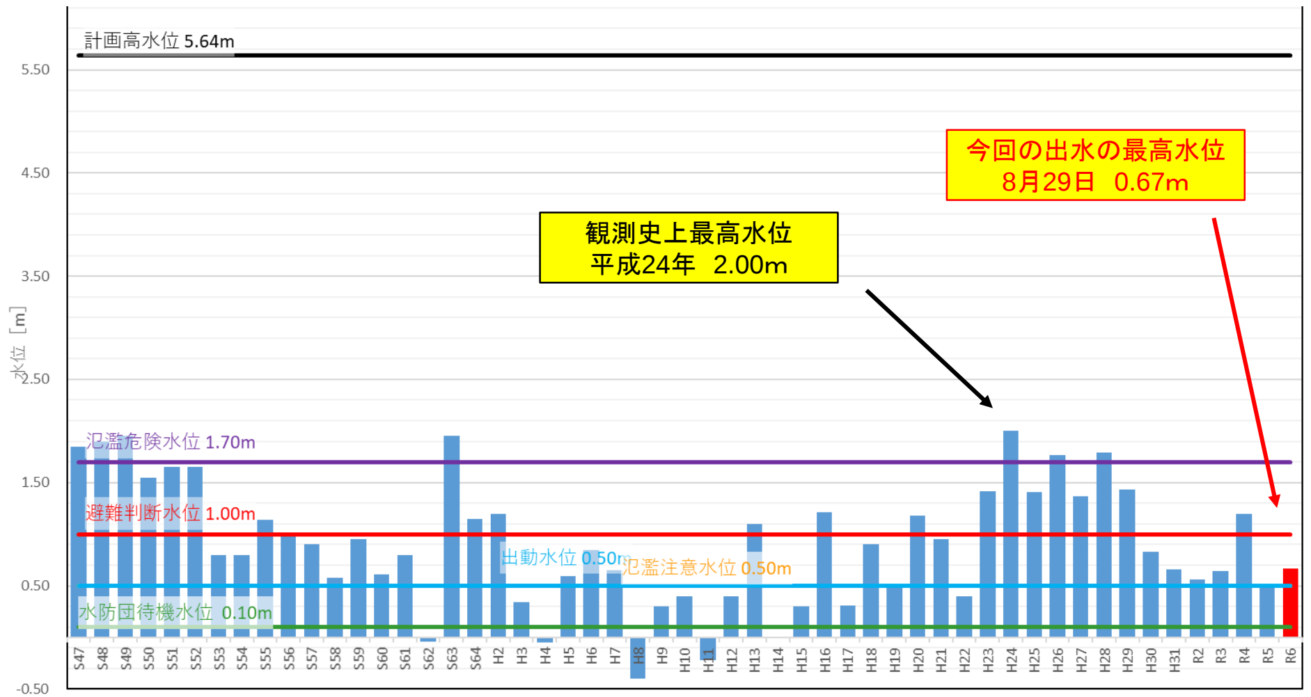
安楽川（川崎水位観測所）の年最高水位比較図
