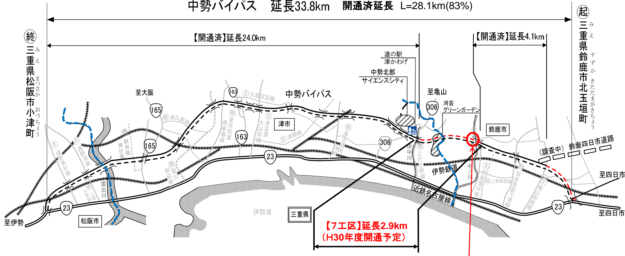
平成29年度23号御園南舗装工事の現場状況 (平成30年10月現在)
