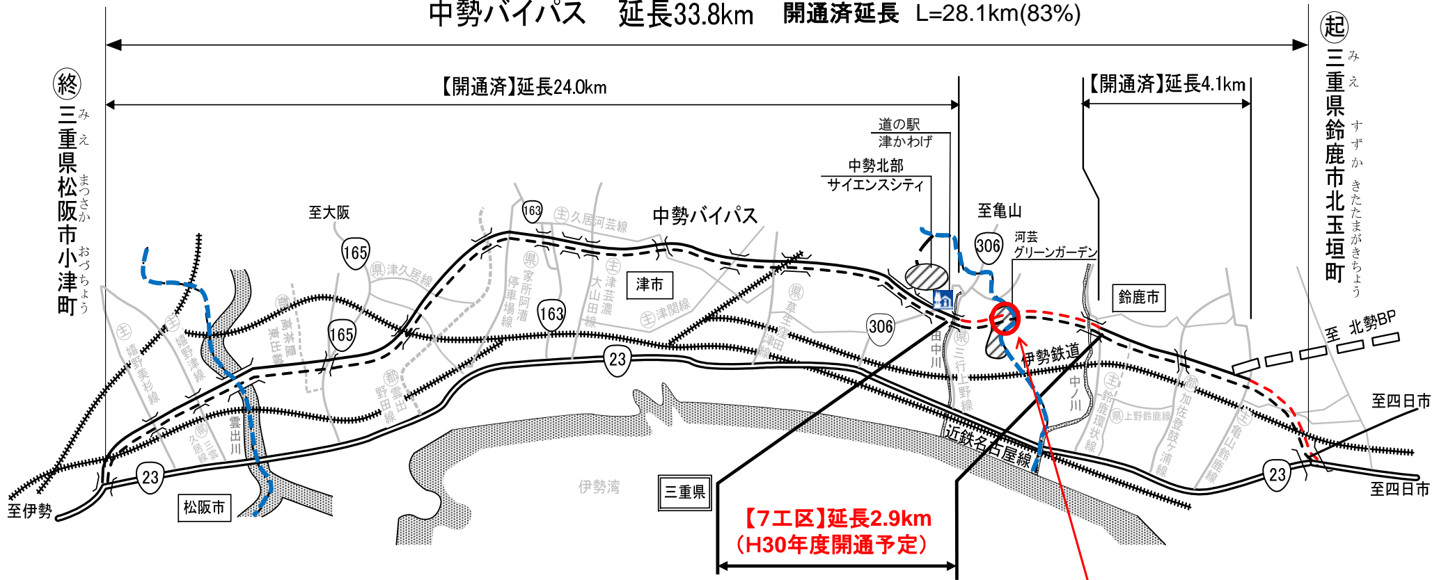
平成29年度23号三行北舗装工事の現場状況 (平成30年9月現在)
