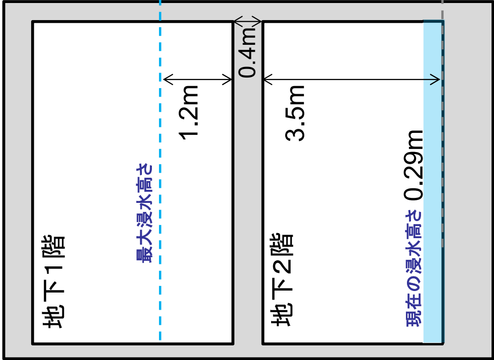
地下駐車場排水進捗状況図(代表点)
