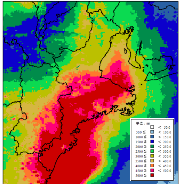
積算降水量分布図 10月21日0時～23日12時 出典:津地方气象台
