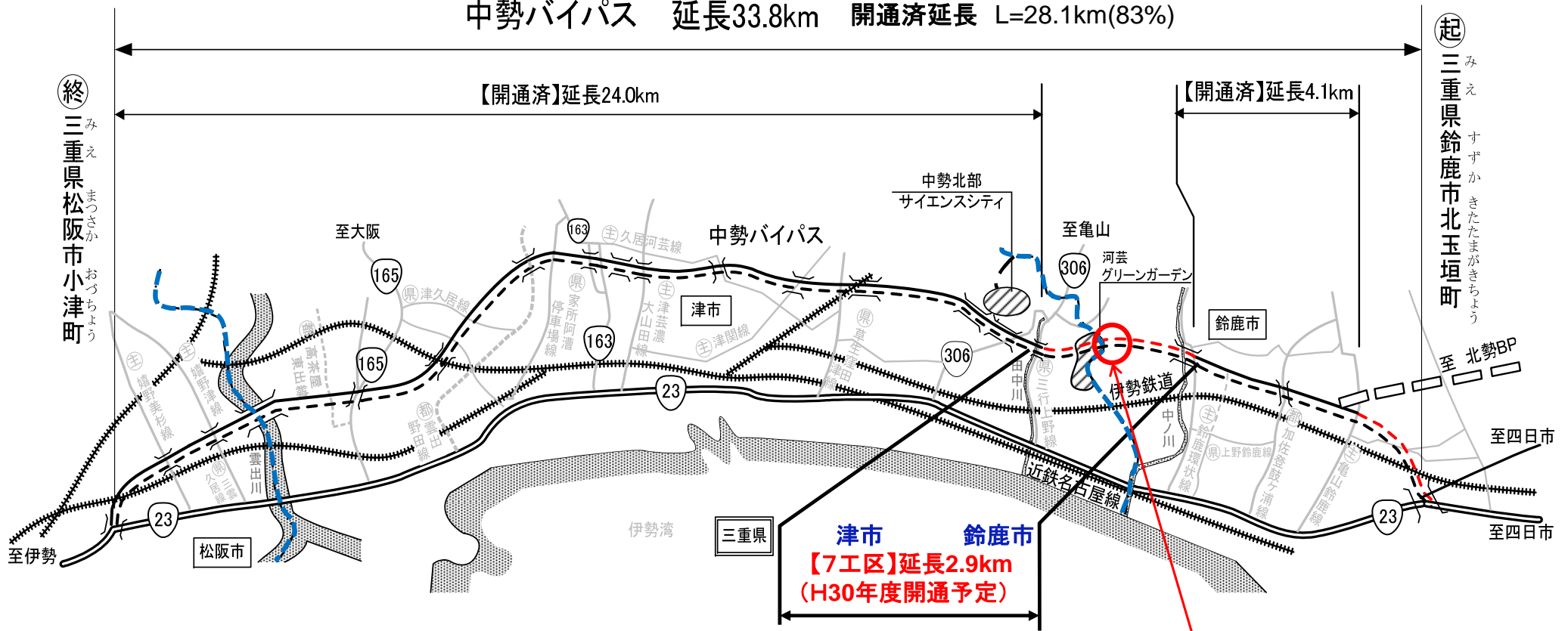
平成28年度23号三行道路建設工事の現場状況 (平成29年9月21日現在)
