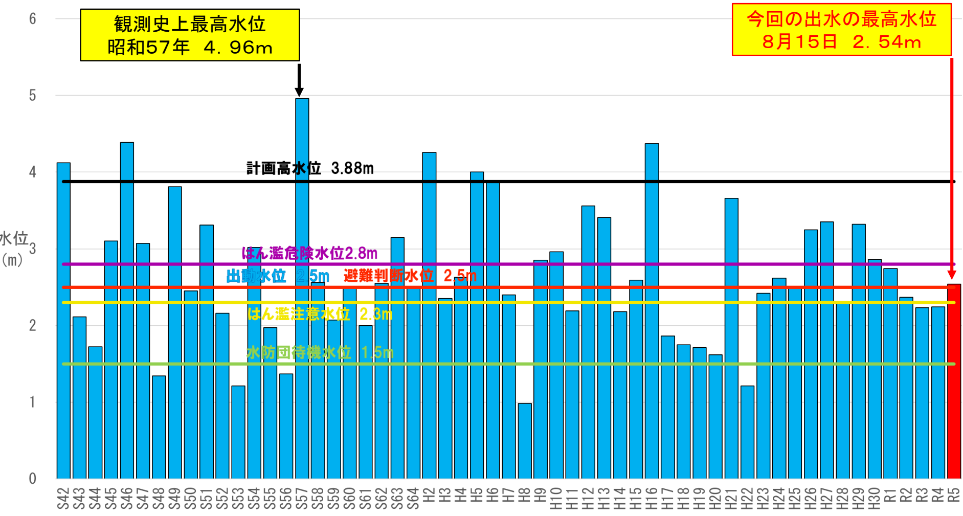
中村川 (島田橋水位観測所) の年最高水位比較図
