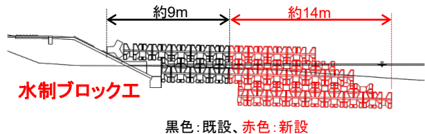
【断面図】A-A'断面
