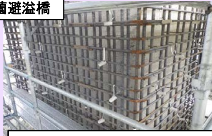
橋脚巻立て 鉄筋組立完了
