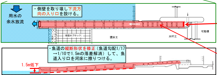
図-5.4 縦断的連続性の再生イメージ (櫛田可動堰)
