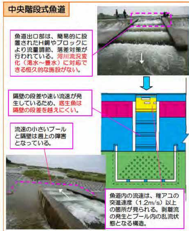
図-3.3 (1) 堰・頭首工の魚道及び河道状況の課題（新屋敷取水堰（東黒部頭首工））
