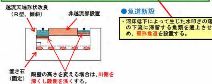
図-5.2 縦断的連続性の再生イメージ（楯田第二頭首工）
