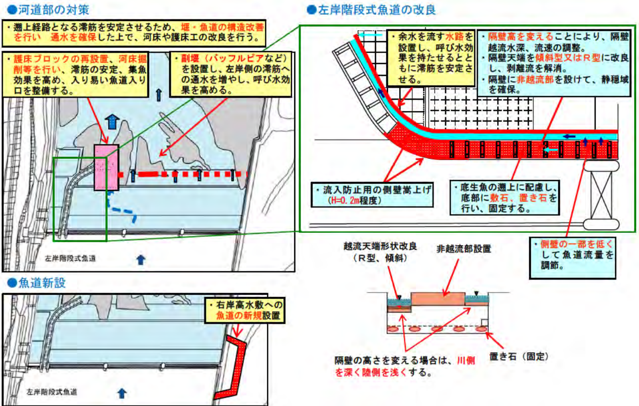
図-5.3 縦断的連続性の再生イメージ（櫛田第一頭首工）
