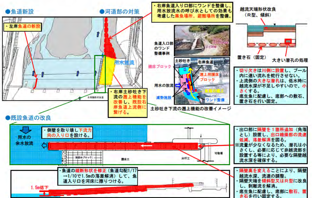
図-5.4 縦断的連続性の再生イメージ（櫛田可動堰）
