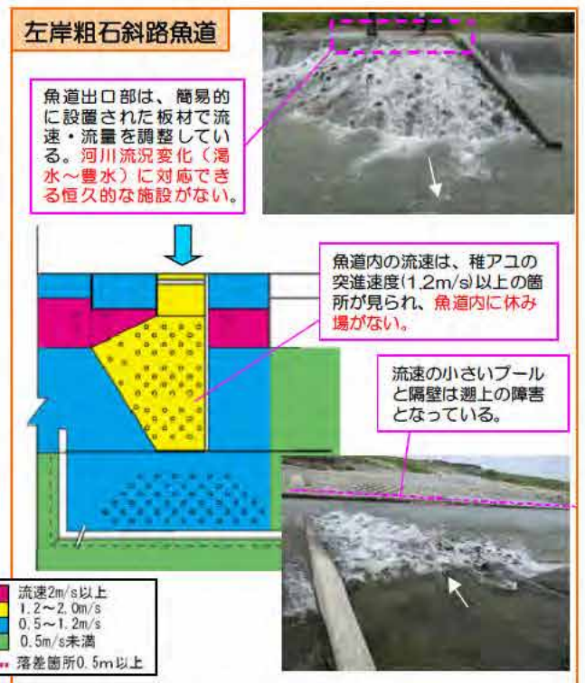
図-3.3 (1) 堰・頭首工の魚道及び河道状況の課題（新屋敷取水堰（東黒部頭首工））
