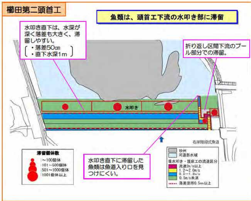
折り返し部の高落差、速い流速部を越えできず途中のプールに滞留する個体が多い。
