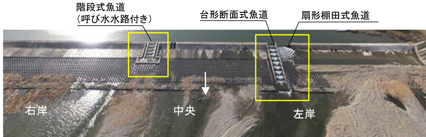
改良：階段式魚道(呼び水水路付き)
