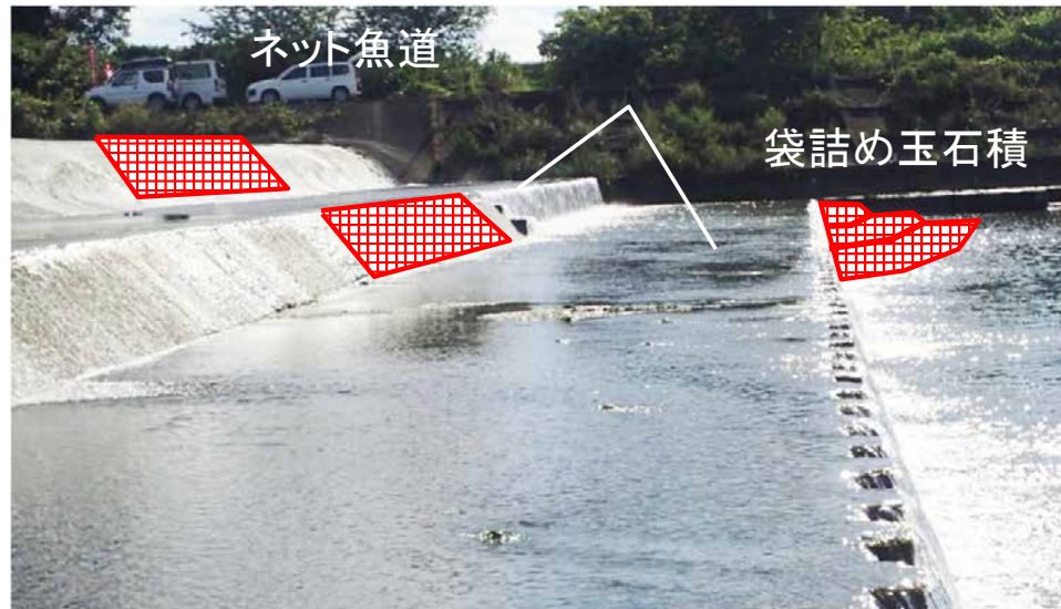
図5-2 仮設ネット魚道と袋詰め玉石積の設置案のイメージ
