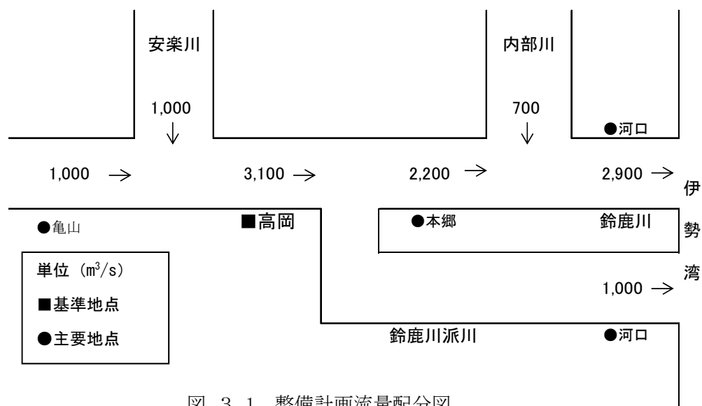
図 3.1 整備計画流量配分図
