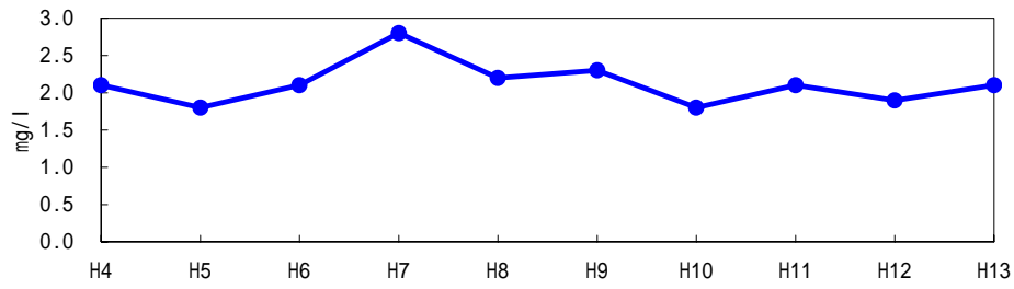
COD(年75%値)
