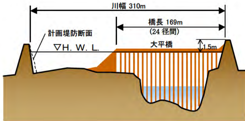
図 2-1-8 大平橋横断面
