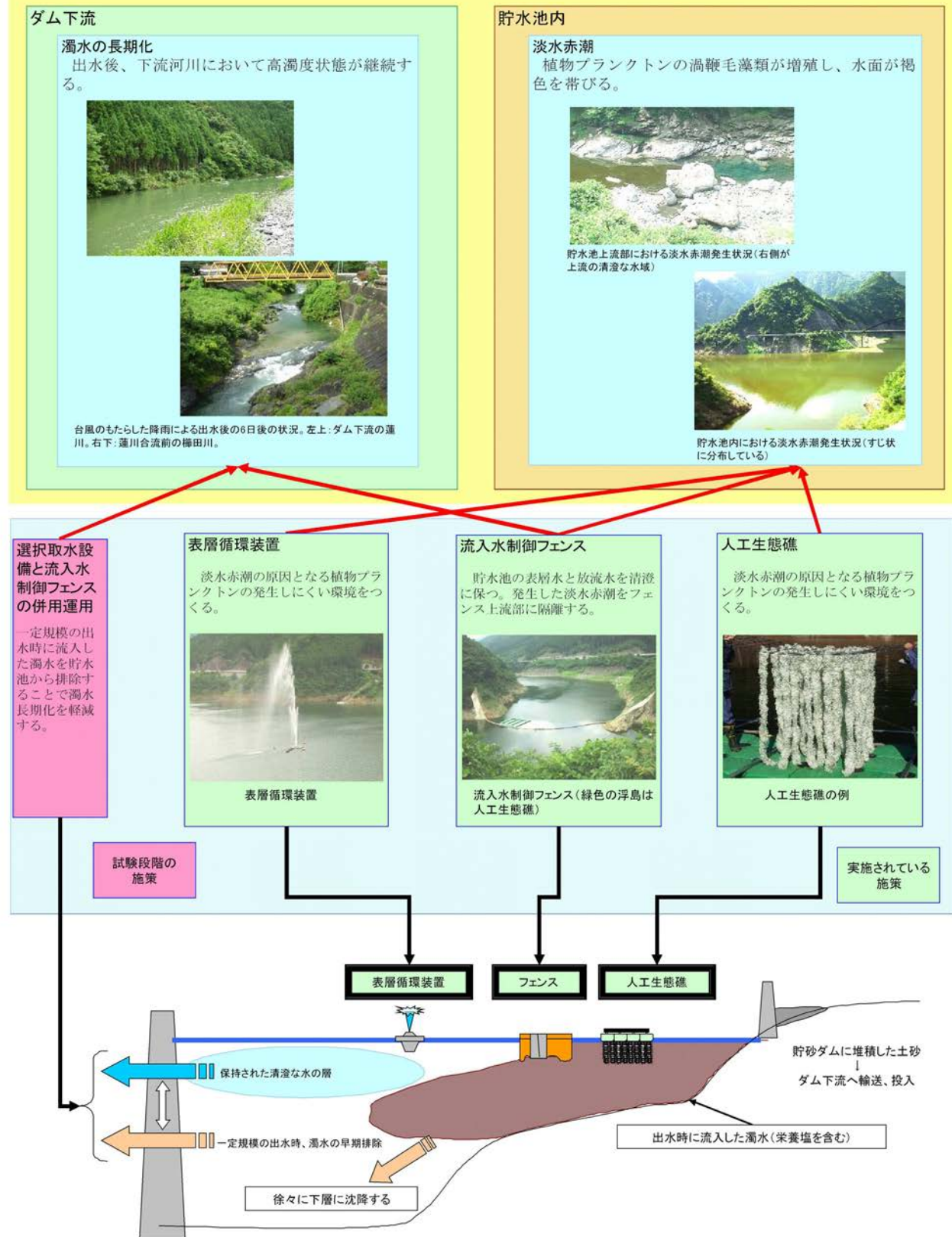
図 2-1-25 連ダムにおける水質問題と対策の実施状況
