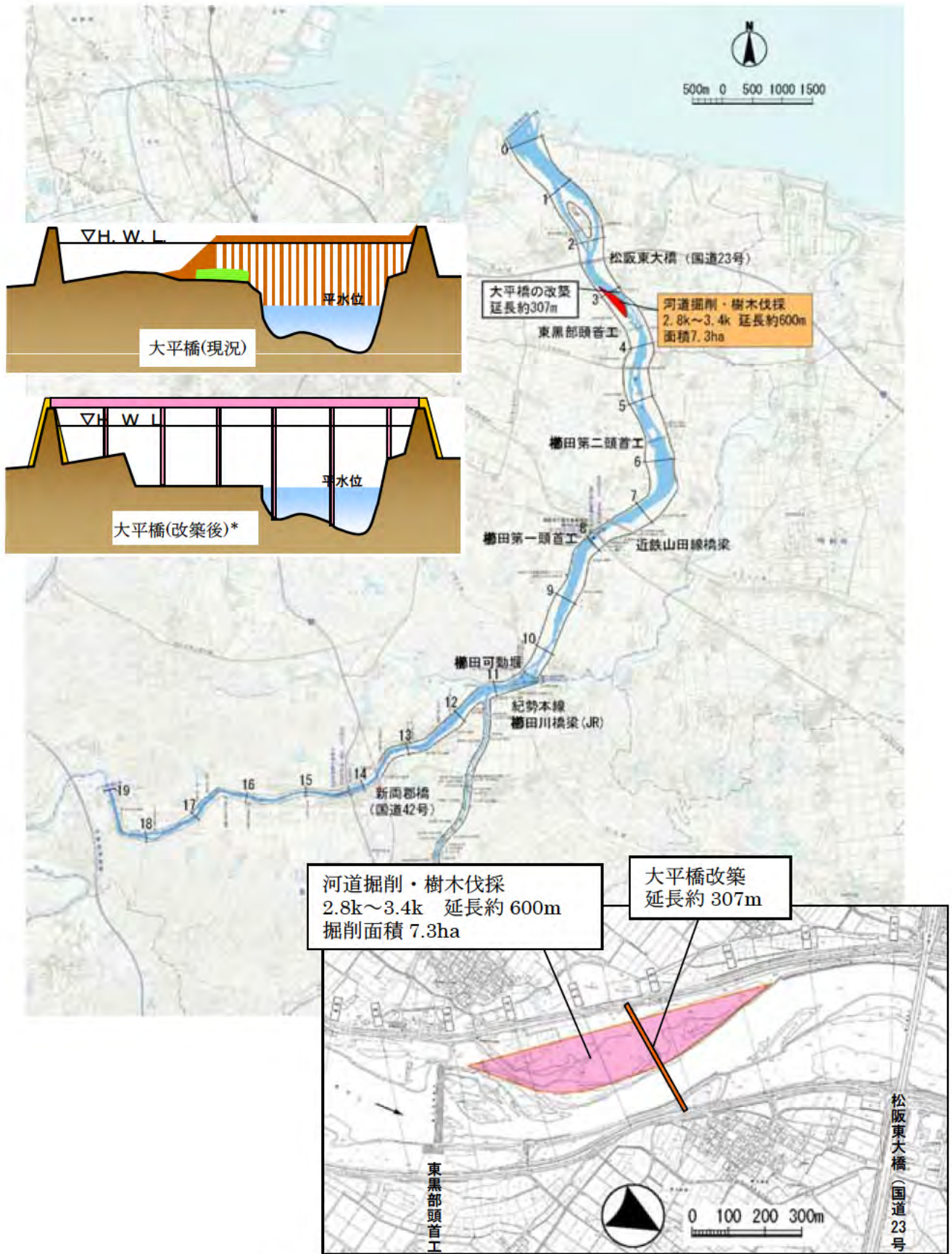
図 4-2-2 水位低下対策位置図とイメージ横断面図 (河道掘削、樹木伐採、大平橋改築)
