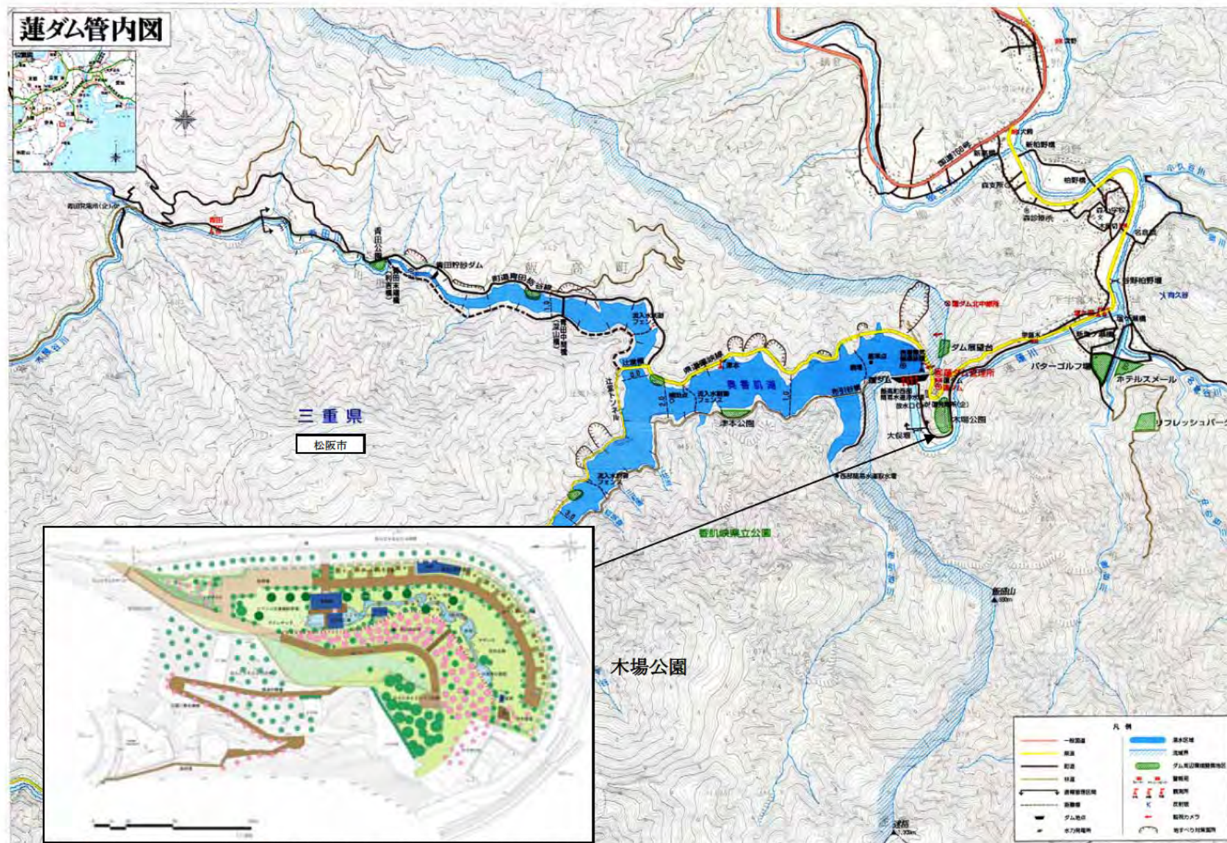
図 4-2-14 蓮ダムの周辺環境整備
