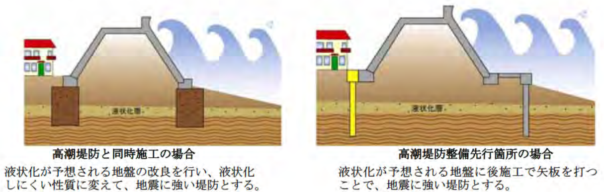
図 4-2-11 耐震対策のイメージ
