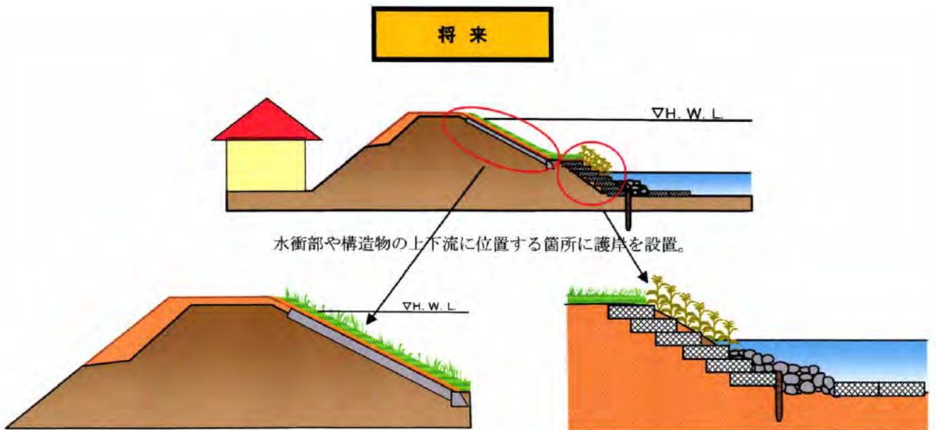
図 4-2-5 高水護岸整備のイメージ
