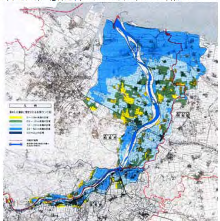
図 4-3-11 楠田川浸水想定区域図 (平成14年1月告示・公表)
