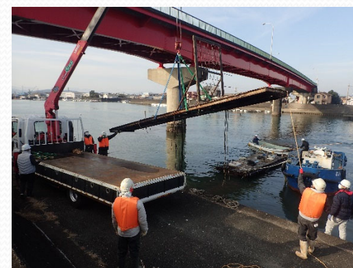
簡易代執行による不法設置栈橋の撤去(令和3年12月実施)
