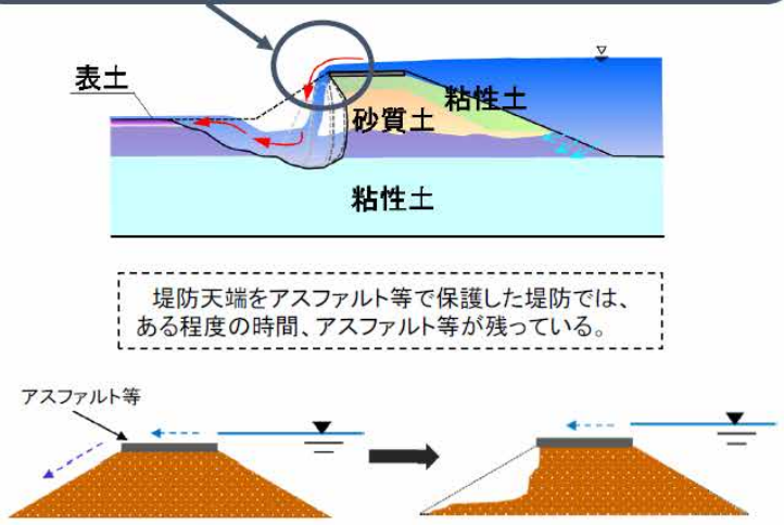
堤防天端の保護 【H32年度まで】
