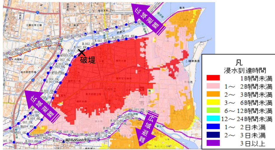
浸水到達時間の事例（鈴鹿川右岸3k地点で破堤した場合）
