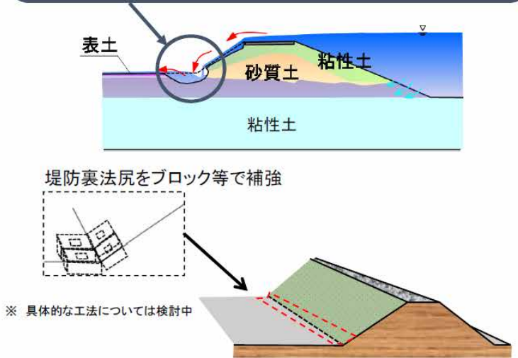
堤防裏法尻の補強 【H32年度まで】
