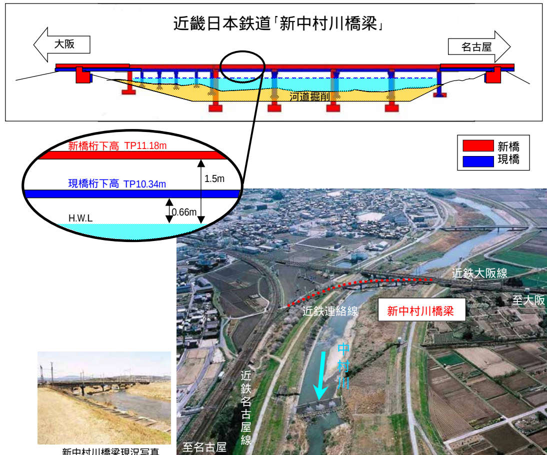
近鉄新中村川橋梁の改築
