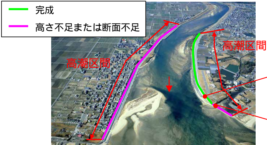
高潮区間と高潮堤防整備状況（雲出川）
