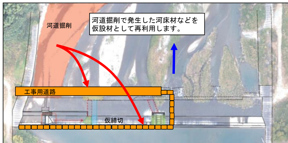
掘削土砂の仮設材としての再利用（イメージ）
