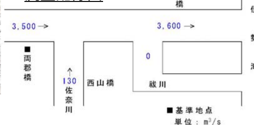
流量配分図
