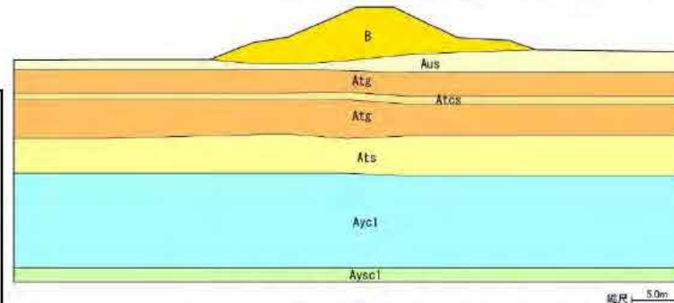
堤防断面の地質 (鈴鹿川左岸2.2k)
