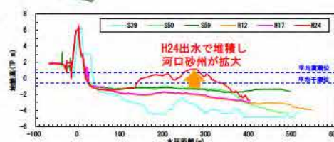
横断変遷 (鈴鹿川0.2km)
