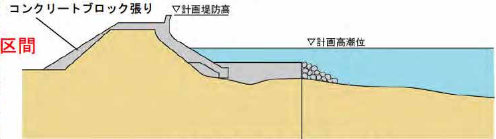
高潮堤防整備イメージ
