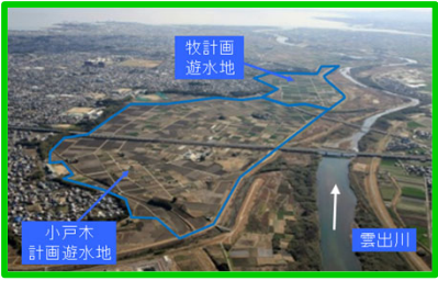
営農機能等を維持した遊水地整備（三重河川国道事務所）
