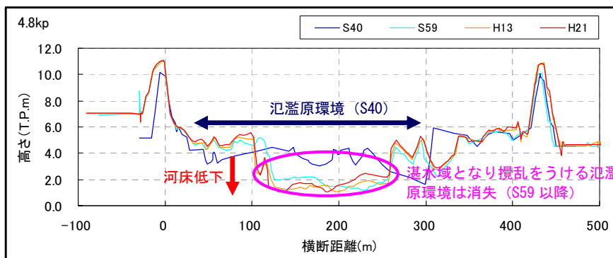
図-2.7 横断面形状の変化にみる氾濫原環境の消失状況 (4.8k)
