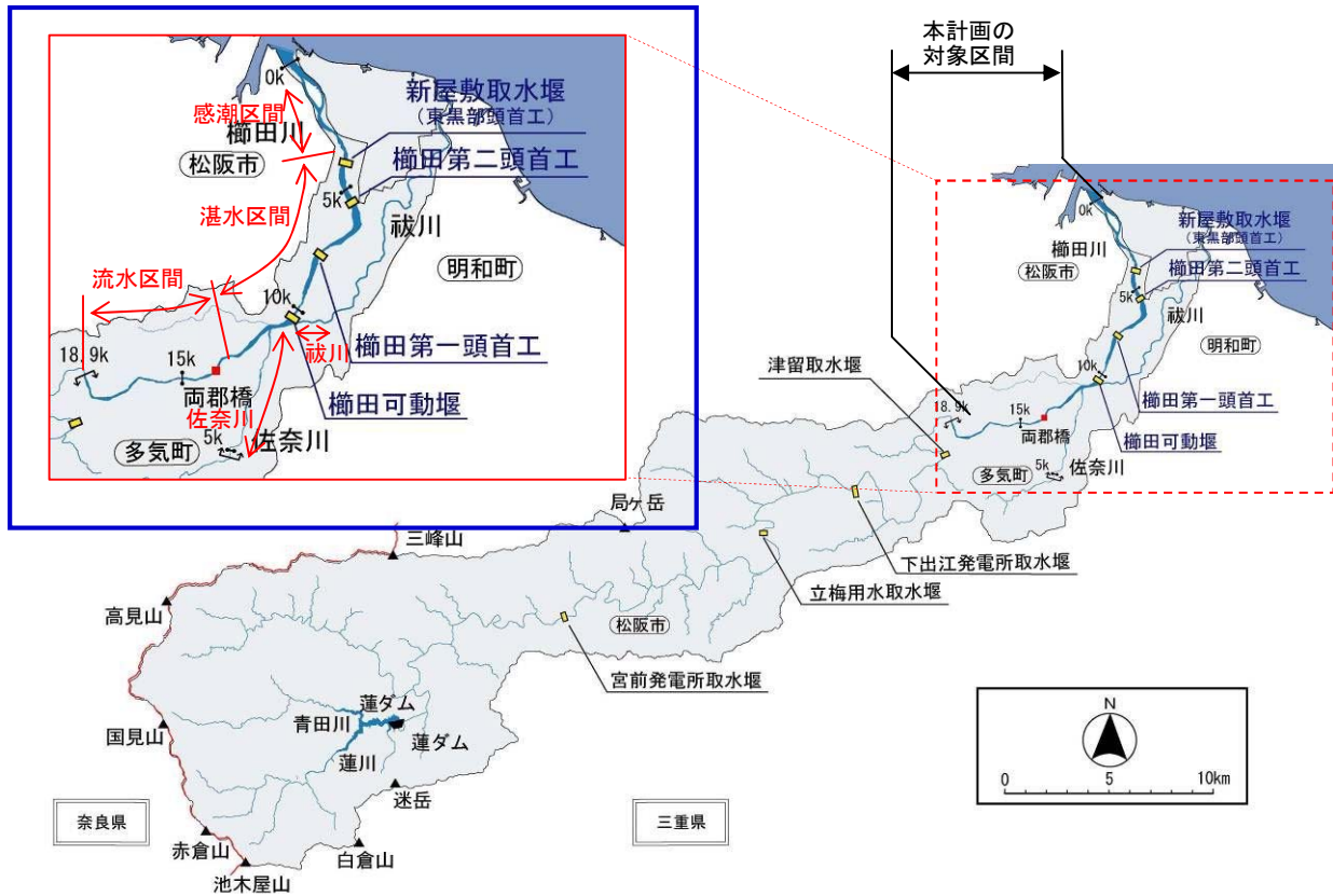
図-2.1 櫛田川流域の河道特性区分
