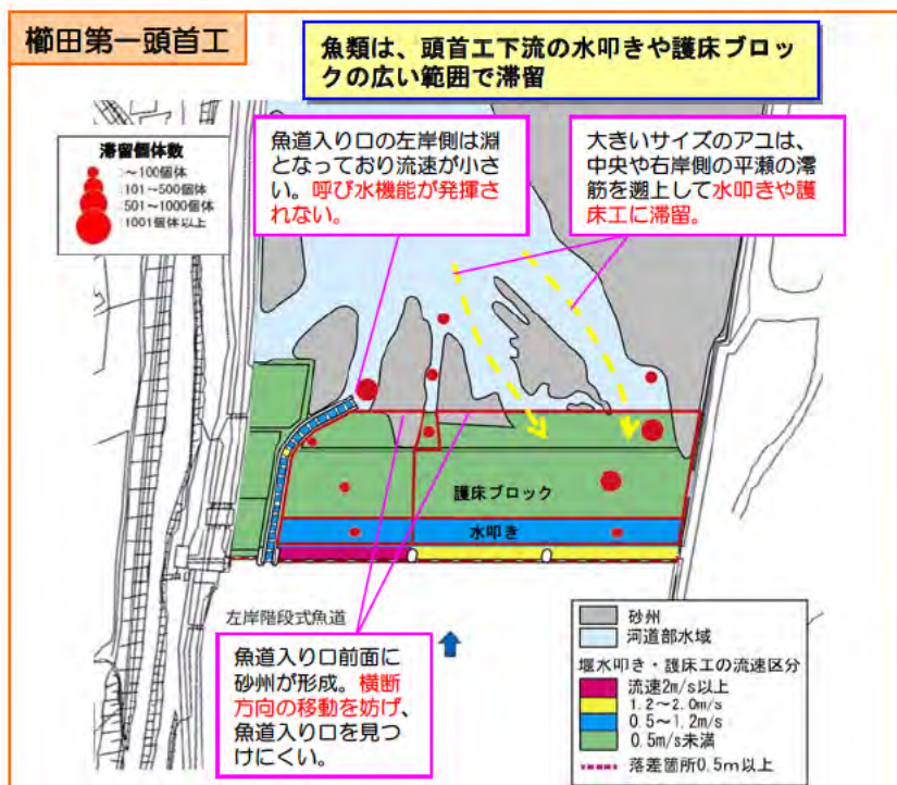
護床工から河道部に砂州が形成し、4つの滞筋をつくり魚類の横断方向の移動を分断。砂州には、樹木が繁茂し始めている。
