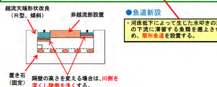
図-5.2 縦断的連続性の再生イメージ（柳田第二頭首工）
