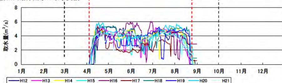
図-2.9 流況の変遷
