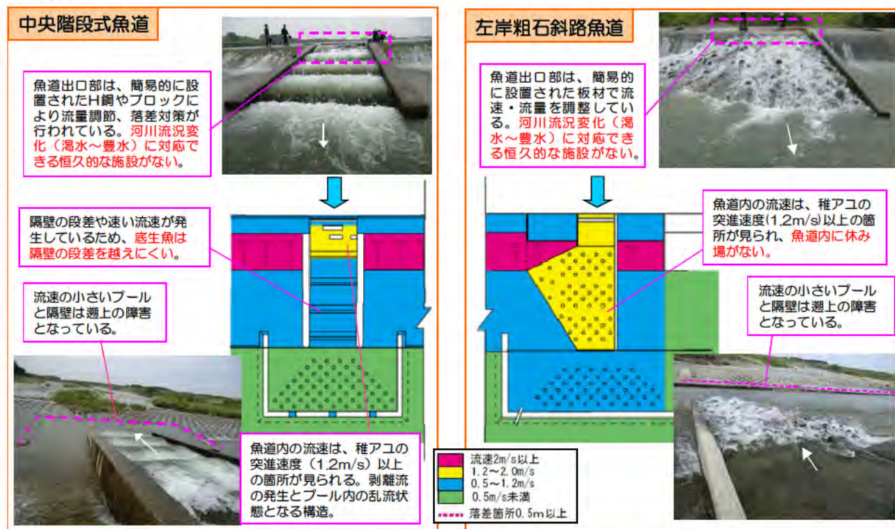
図-3.3 (1) 堰・頭首工の魚道及び河道状況の課題（新屋敷取水堰（東黒部頭首工））
