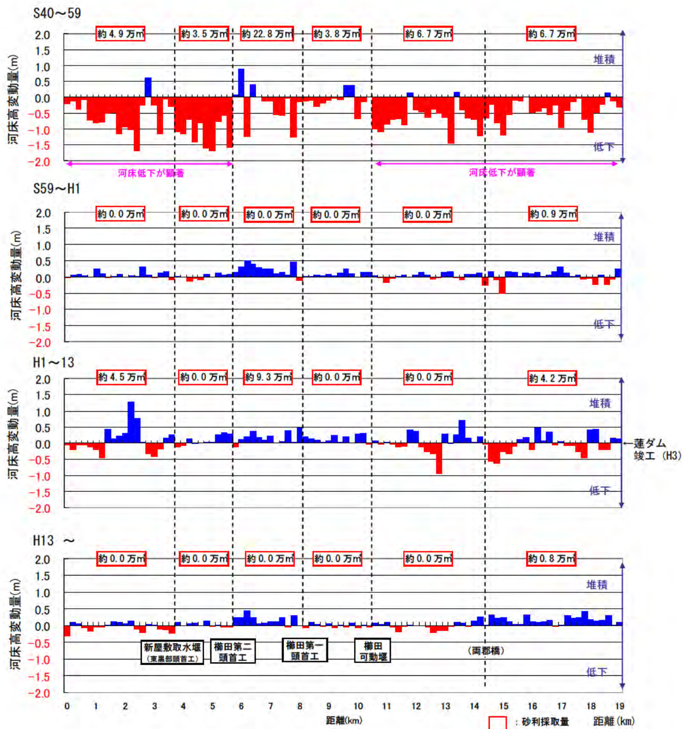
図-2.4 期間別の平均河床高変動量
