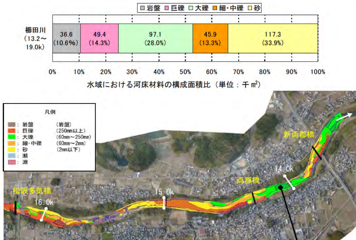
図-2.19 新両郡橋～松阪多気橋付近の河床材料分布図 (H24 現地調査結果による)
