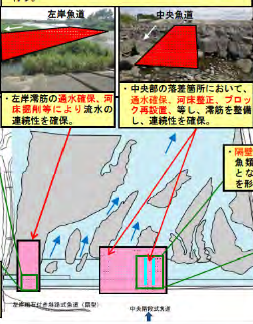
図-5.1 縦断的連続性の再生イメージ（新屋敷取水堰）
