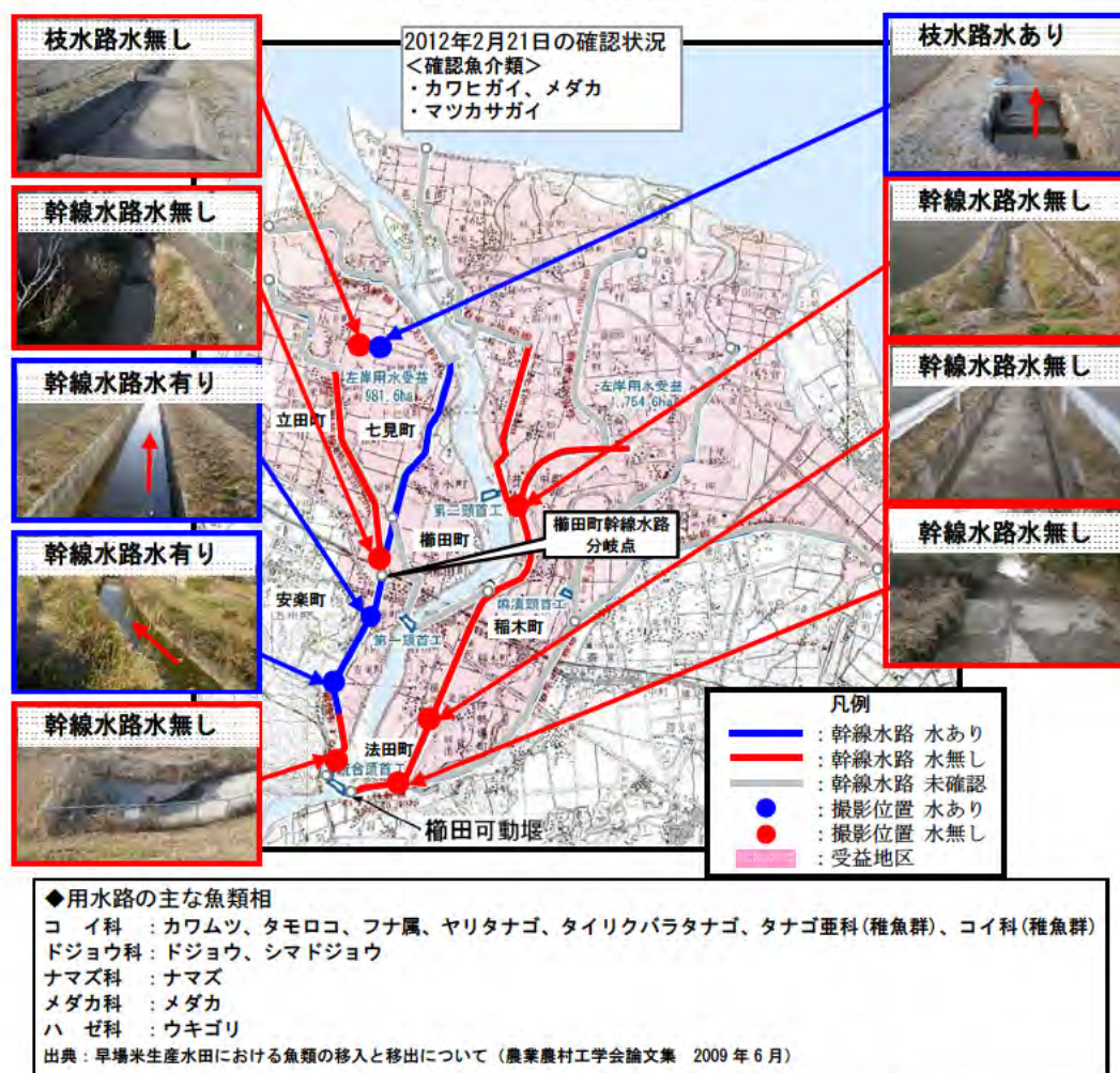
図-2.31 櫛田可動堰下流の用水路網と水溜まり、水枯れ状況
