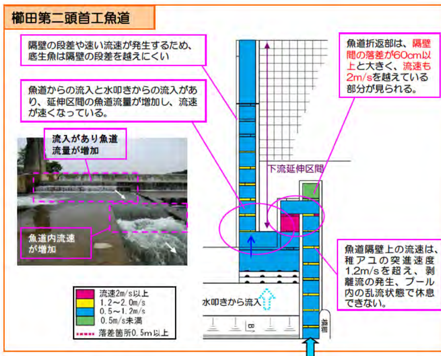
図-3.3 (2) 堰・頭首工の魚道及び河道状況の課題（櫛田第二頭首工）
