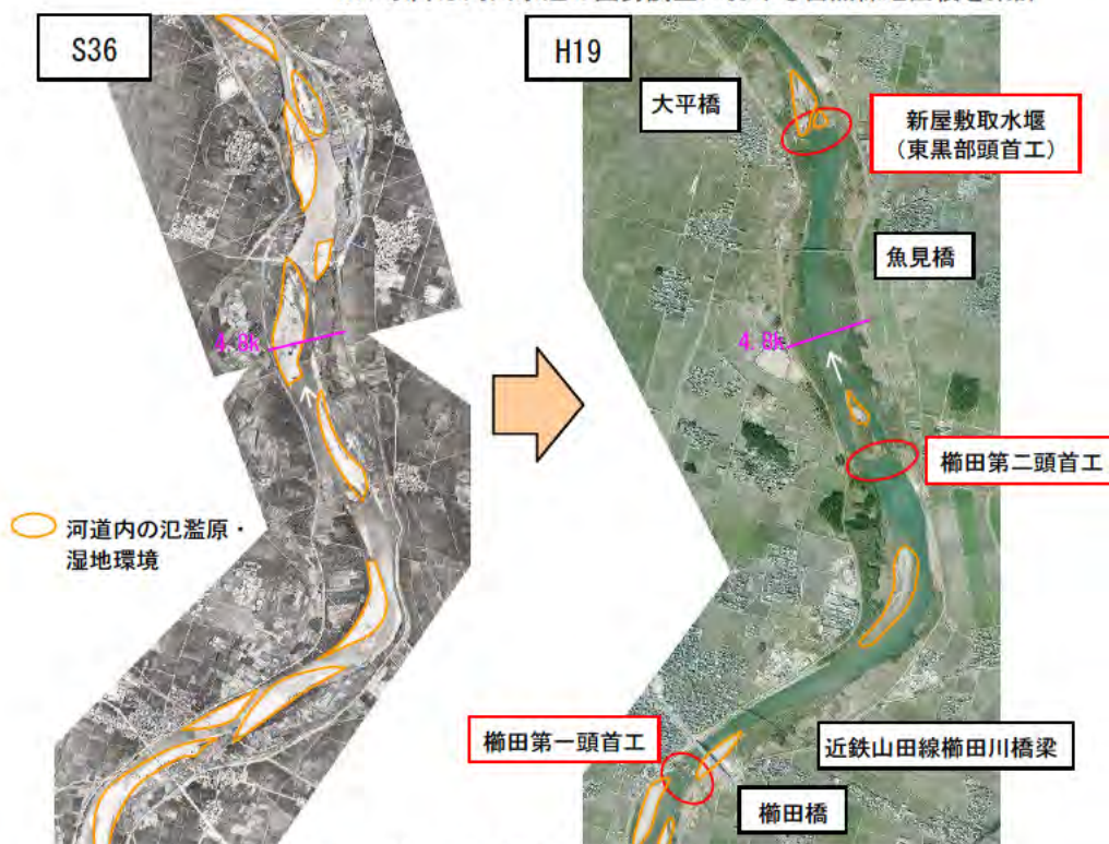
図-2.6 湛水区間における河道内の氾濫原・湿地環境の変遷
