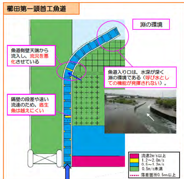
図-3.3 (3) 堰・頭首工の魚道及び河道状況の課題（柳田第一頭首工）
