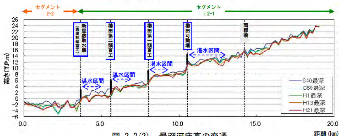
図-2.2(2) 最深河床高の変遷
