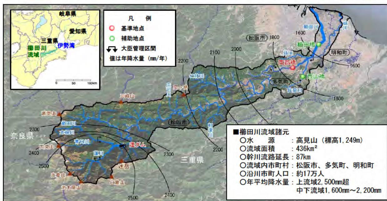
図-1.1 流域図
