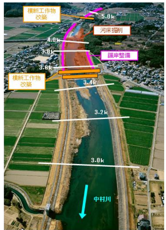
図 35 中村川での河川整備計画に基づく河道整備
