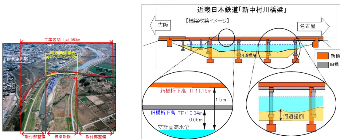
図 23 近畿日本鉄道連絡線新中村川桥梁の特定構造物改築事業の概要
