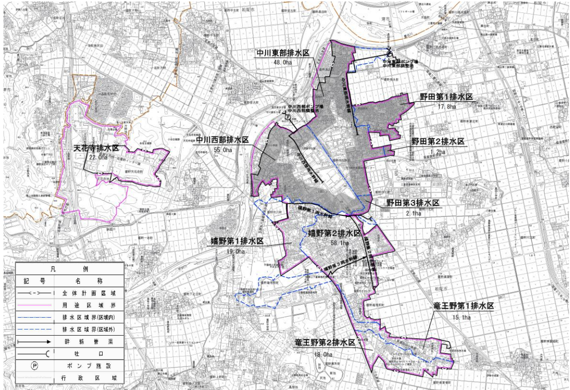
図 14 下水道全体計画区域（嬉野管内）（松阪市公共下水道事業（雨水））
