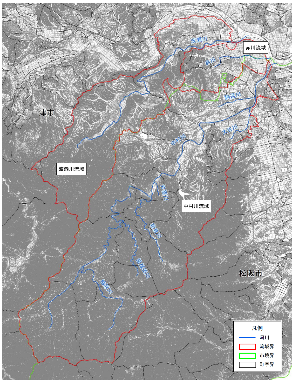
図 28 特定都市河川流域図
