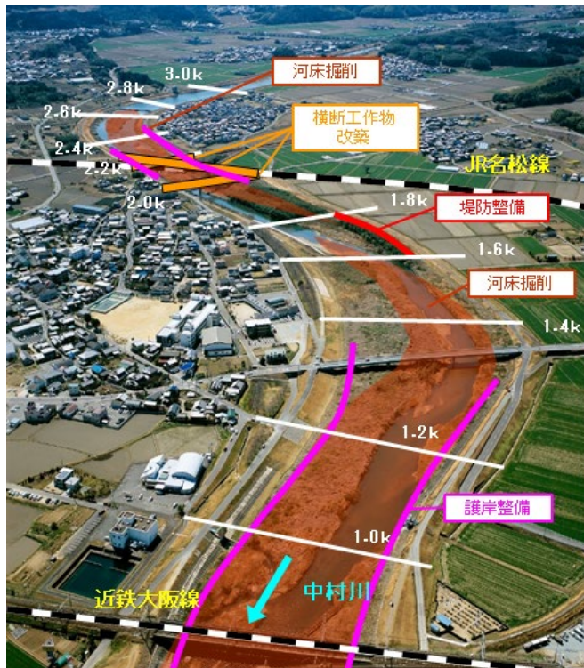
図 32 中村川での河川整備計画に基づく河道整備
