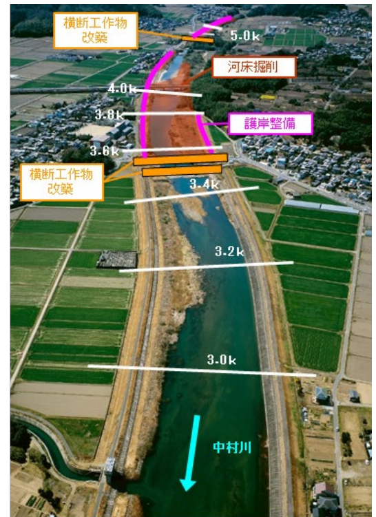
図 32 中村川での河川整備計画に基づく河道整備
