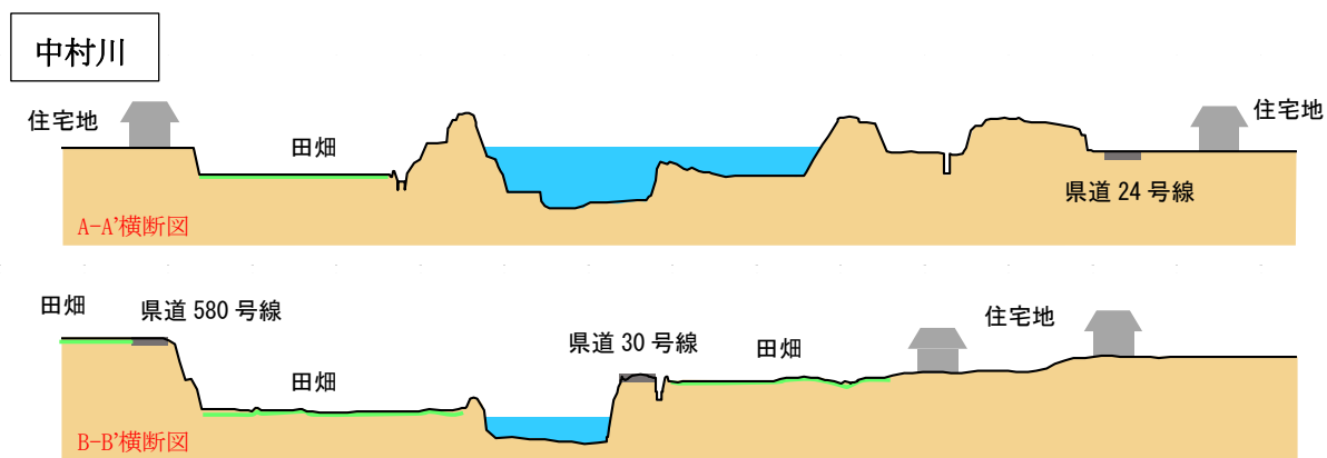
図 3 中村川流域の標高図・代表的な横断面図 (イメージ)
