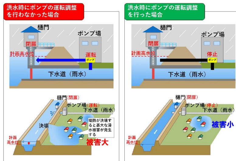
図 41 内水排除ポンプの運転イメージ
