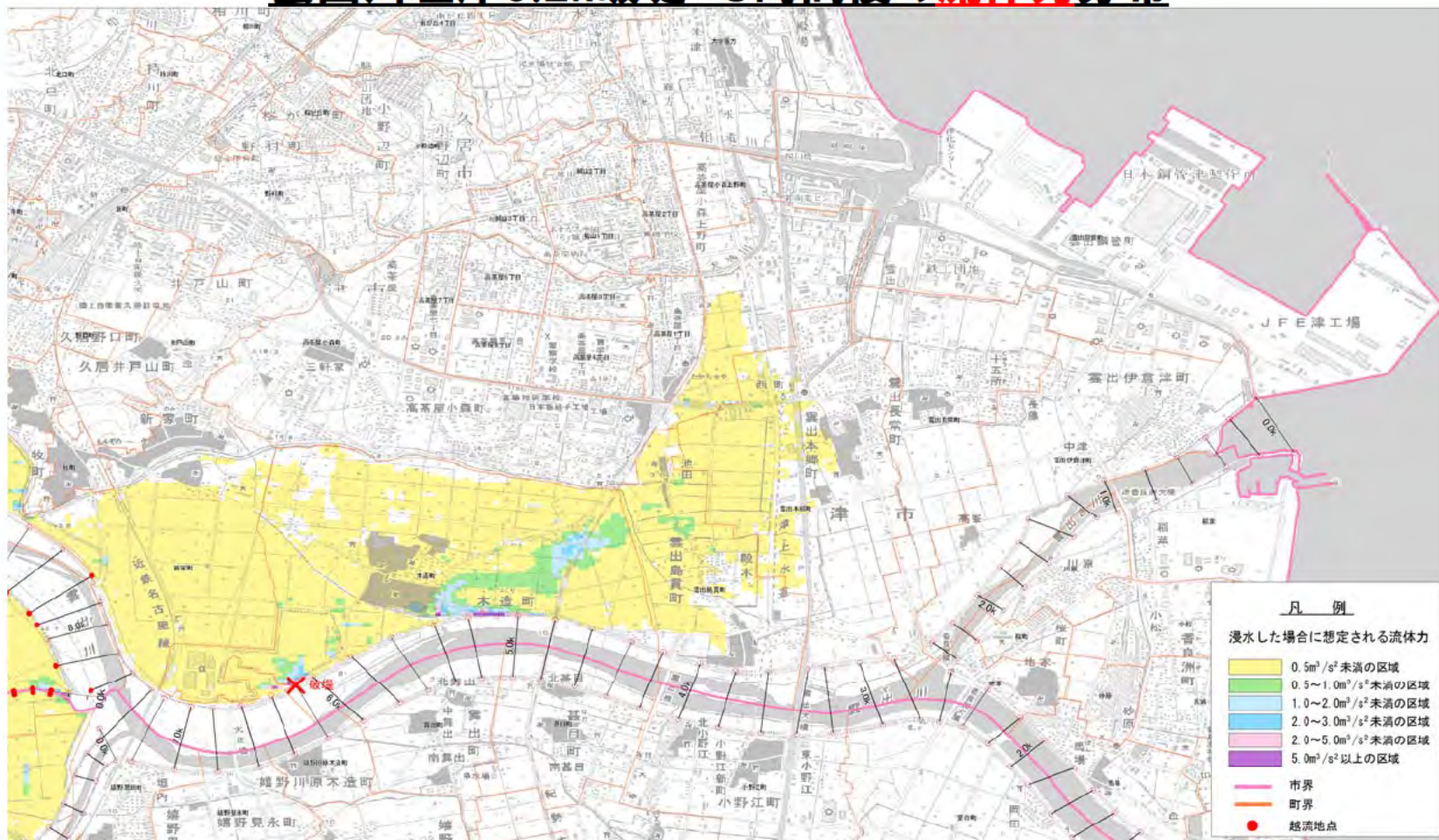
雲出川左岸6.2k破堤 3時間後の流体力分布
