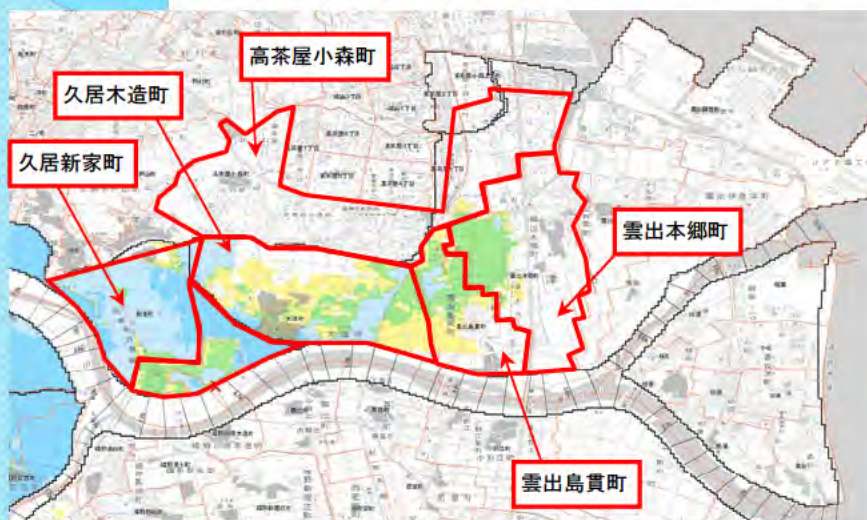
雲出川左岸6.2k破堤 3時間後の被害状況
