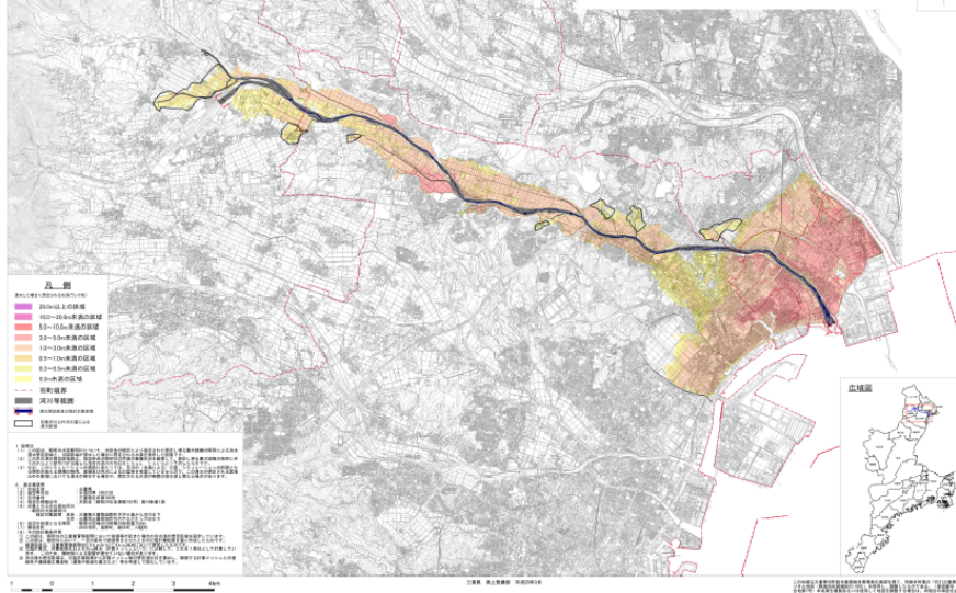
洪水浸水想定区域図（想定最大規模）【朝明川水系】
