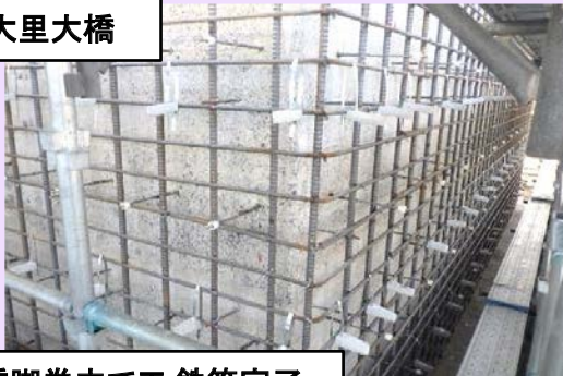
橋脚巻立て工 鉄筋完了
