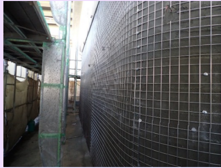
橋脚巻立て工 ラス網設置完了
