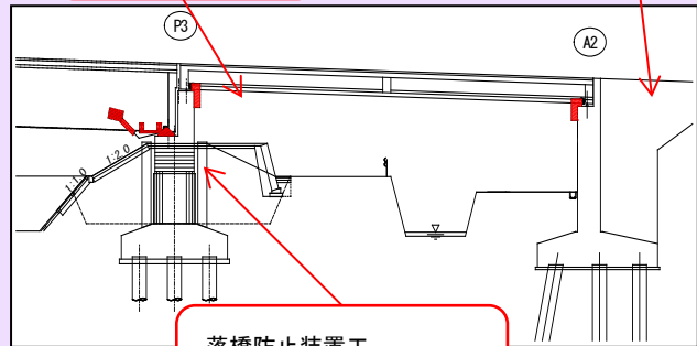
落橋防止装置工 緩衝チェーン・縦型緩衝ピン
