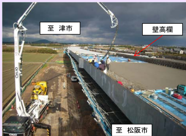
床版コンクリートの打設 施工状況
