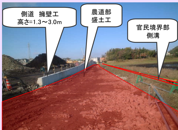
東側
