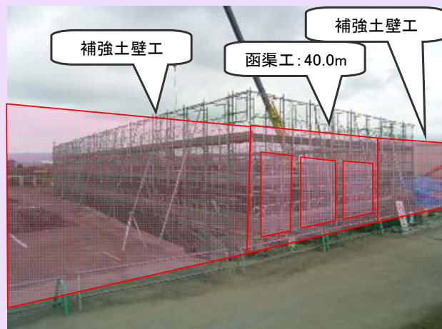
函渠工
