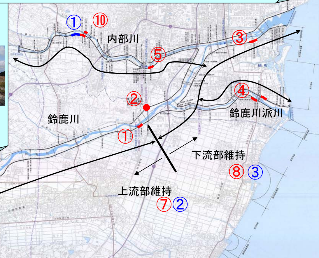
④ 平成22年度 鈴鹿川派川北五味塚高潮堤防工事
